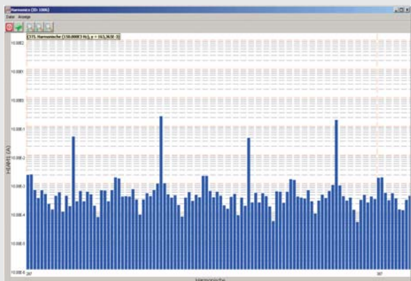
ZES ZIMMER的软件LMG-CONTROL的谐波分析
