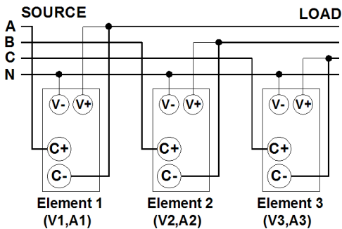
三相 4 线制 (3P4W)
