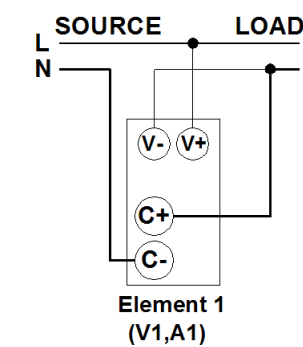
接线图1：不带传感器 单相 2 线制 (1P2W)
