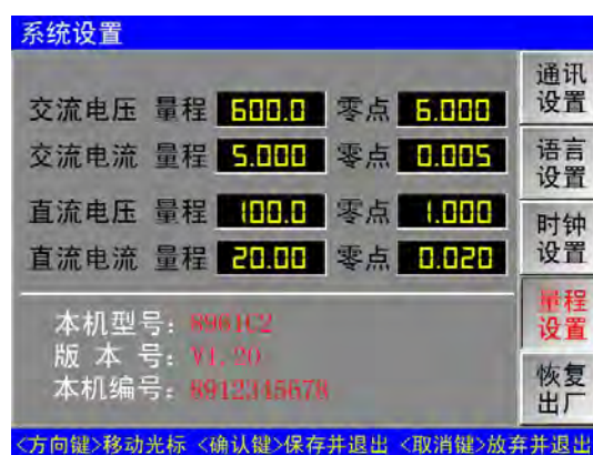
图 14-4 量程设置屏幕
