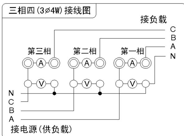
图 4-6 3P4W 接线图
