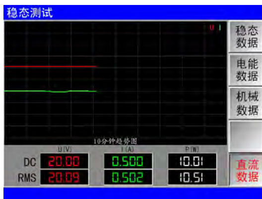
图 5-3 直流数据
