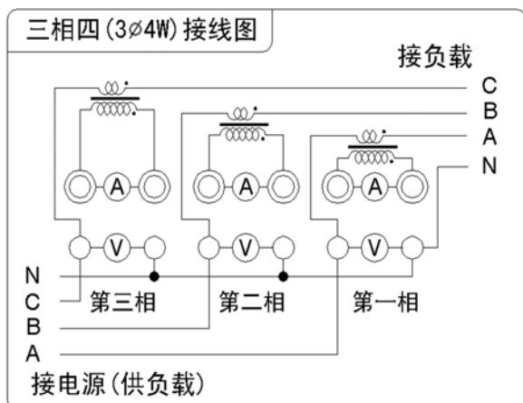
图 4-10 三相四线（3P4W—CT）接线图
