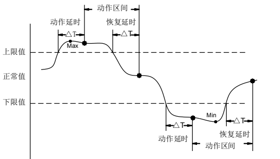
报警输出控制过程示意图
