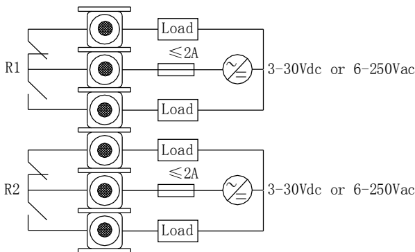
仪表继电器输出典型接线图
