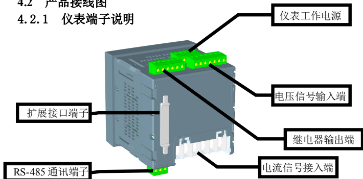
仪表输入输出端子位置示意图
