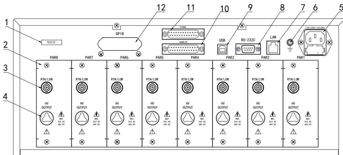
图 3-2 后面板说明
