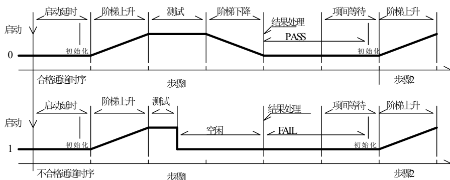
仪器测试时序示意图 (2017.10 修改)
