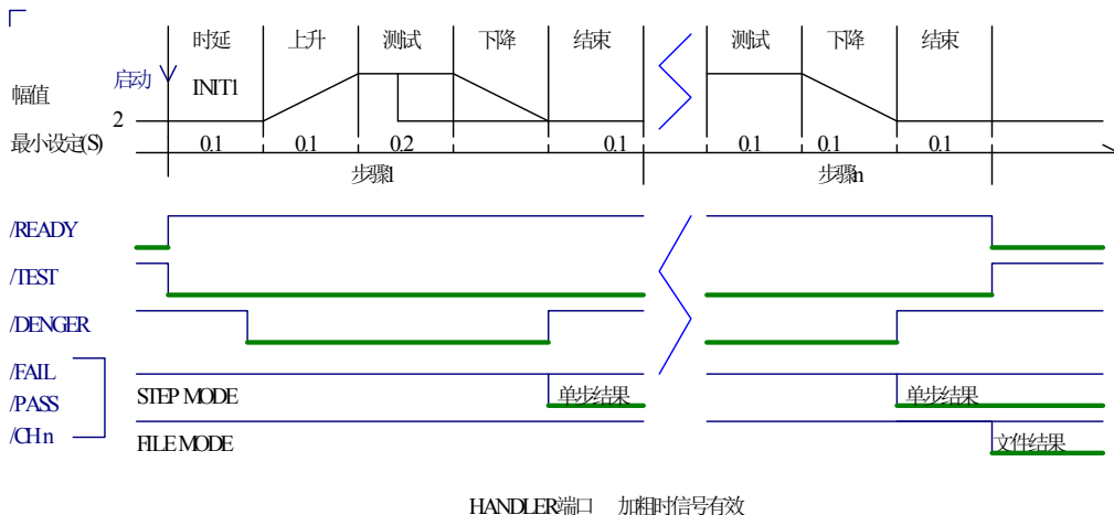
图 4.5.2: HANDLER 接口时序示意视图
