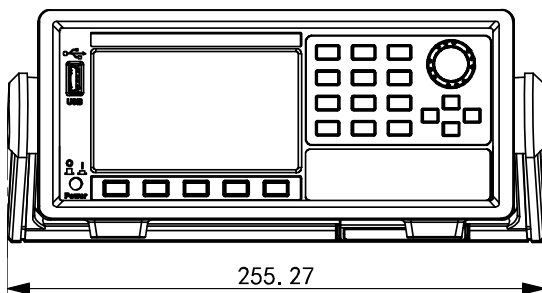
详细尺寸图
