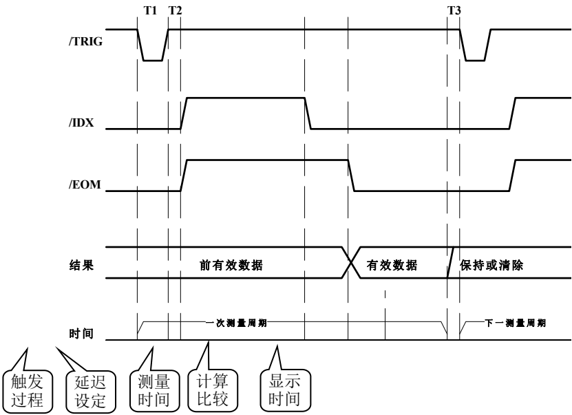
图 5-2 接口信号的时序图
