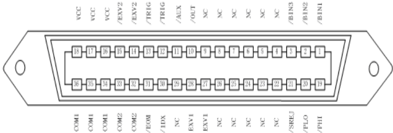
图 5-1 Handler 接口管脚定义
