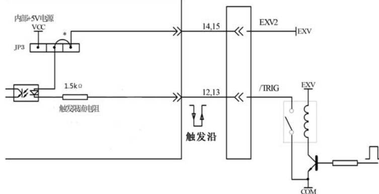
图 5—6 用继电器控制触发
