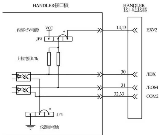
图 5-4 控制输出信号简化示意图
