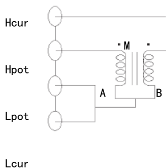
图 6—4 互感直接测量法
