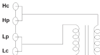
图 6—6 变压器绕组间电容测量
