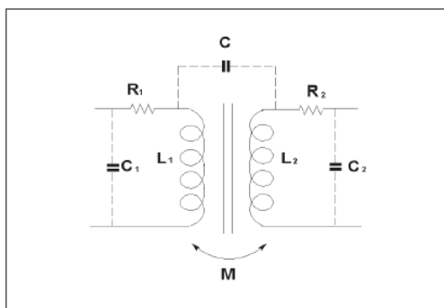
图 6—1 变压器及其参数示意
