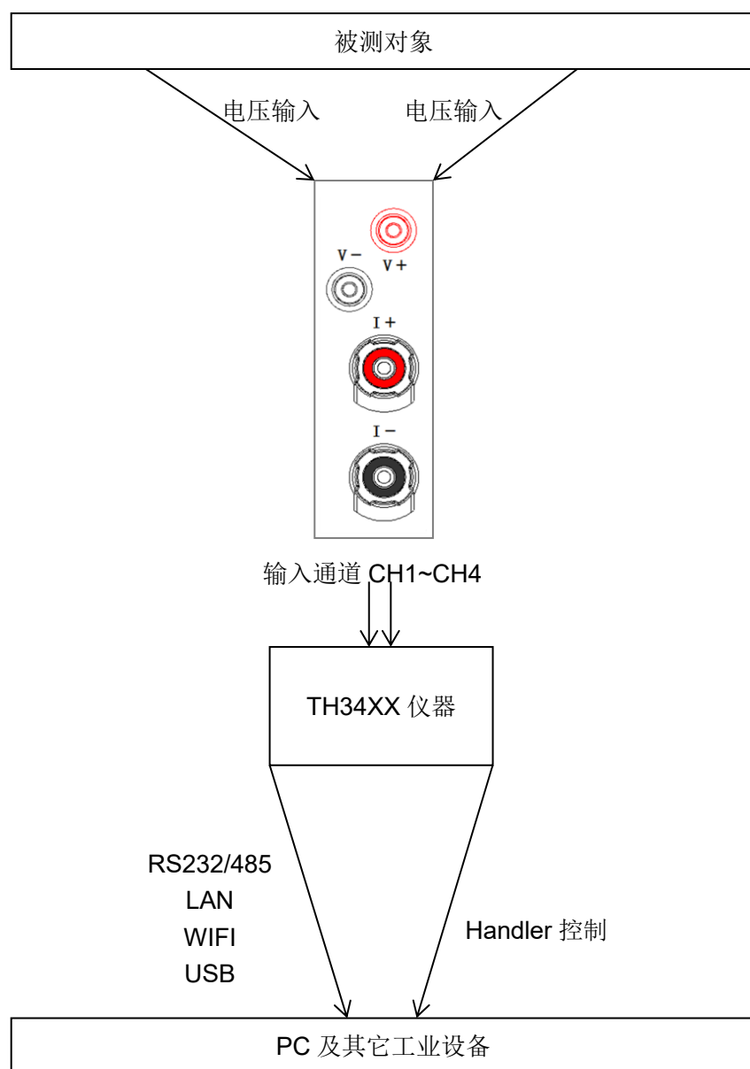
(图 9-1 系统构造)
