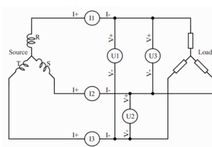
图 8-7 3V3A 示意图
