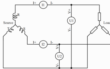
图 8-5 3P3W 示意图
