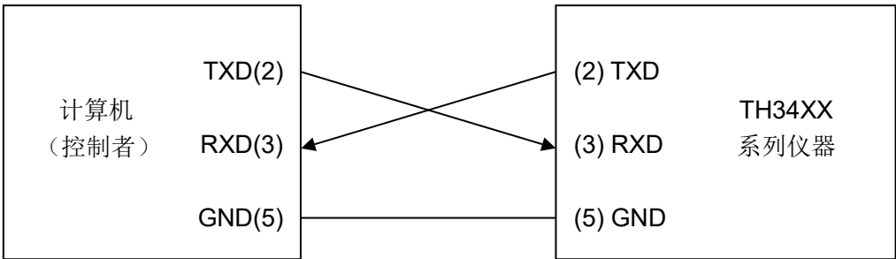
图 10-2 计算机与仪器连接示意图
