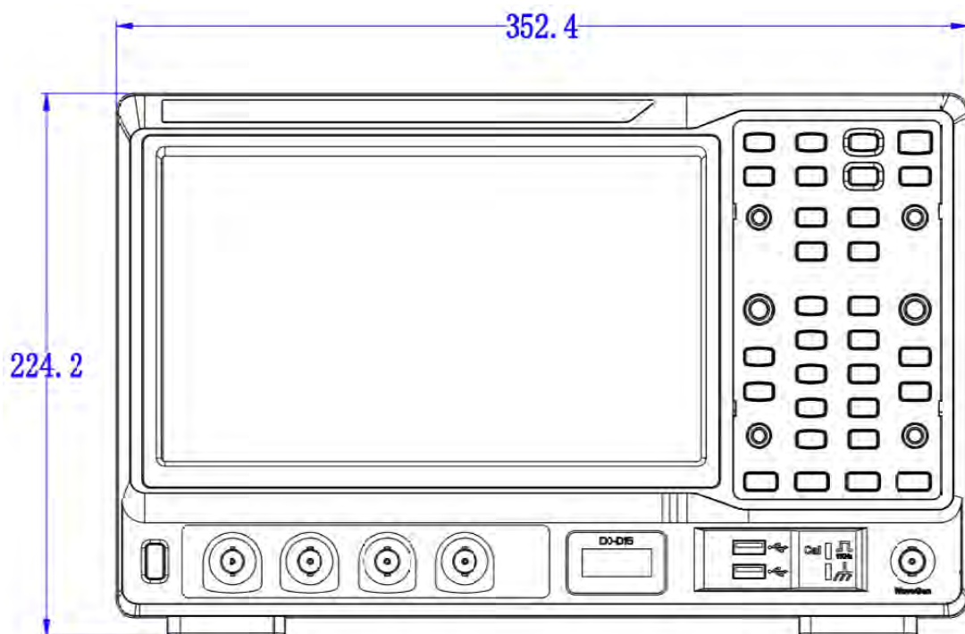
正视图
