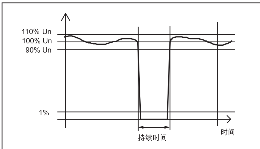
图 15. 电压中断
