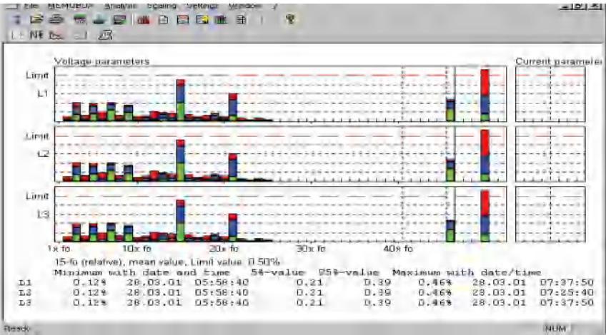
图 22. 电压和电流谐波的累积频率
