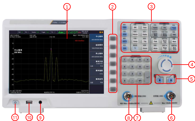
图 4-1 前面板概览
