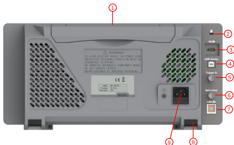
图 4-6 后面板视图
