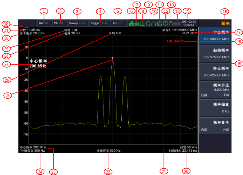
图 4-7 用户界面
