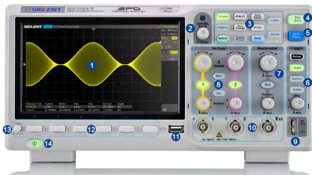
图 8.2 通道机型前面板总览
