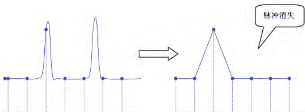
图 28 波形漏失
