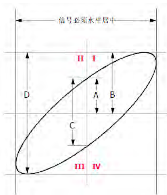
图 20 李沙育测量原理图
