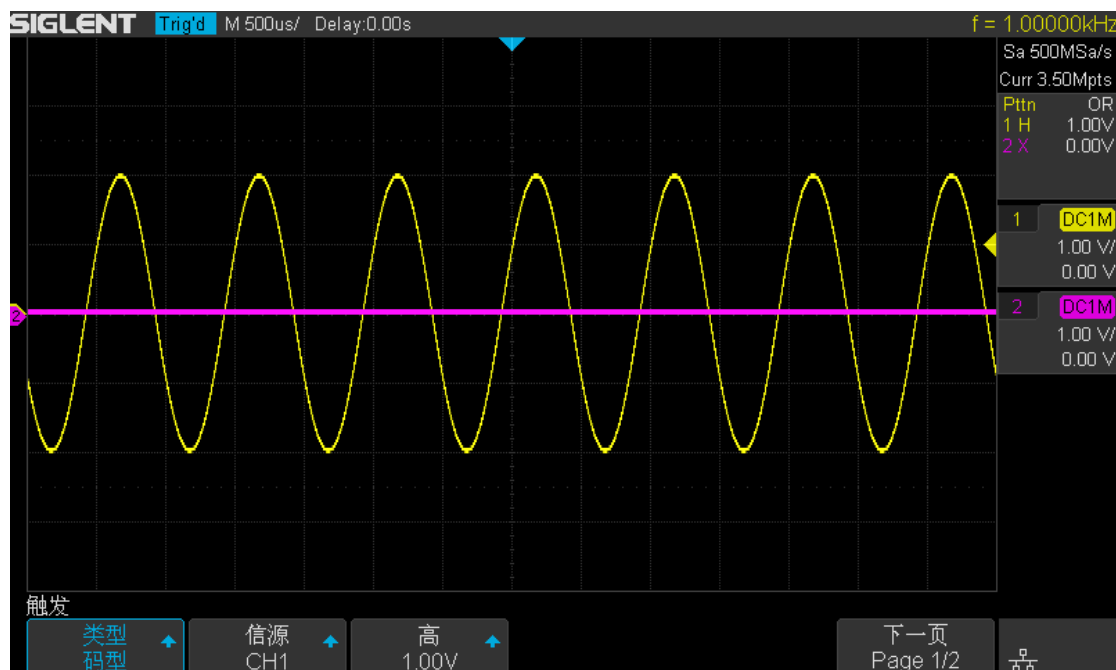
图 49 码型触发 1 (1/2 页)
