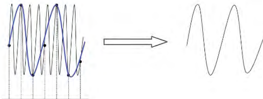
图 27 波形混叠
