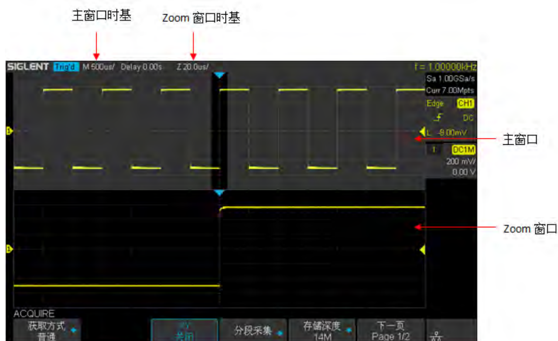
图 22 分屏缩放
