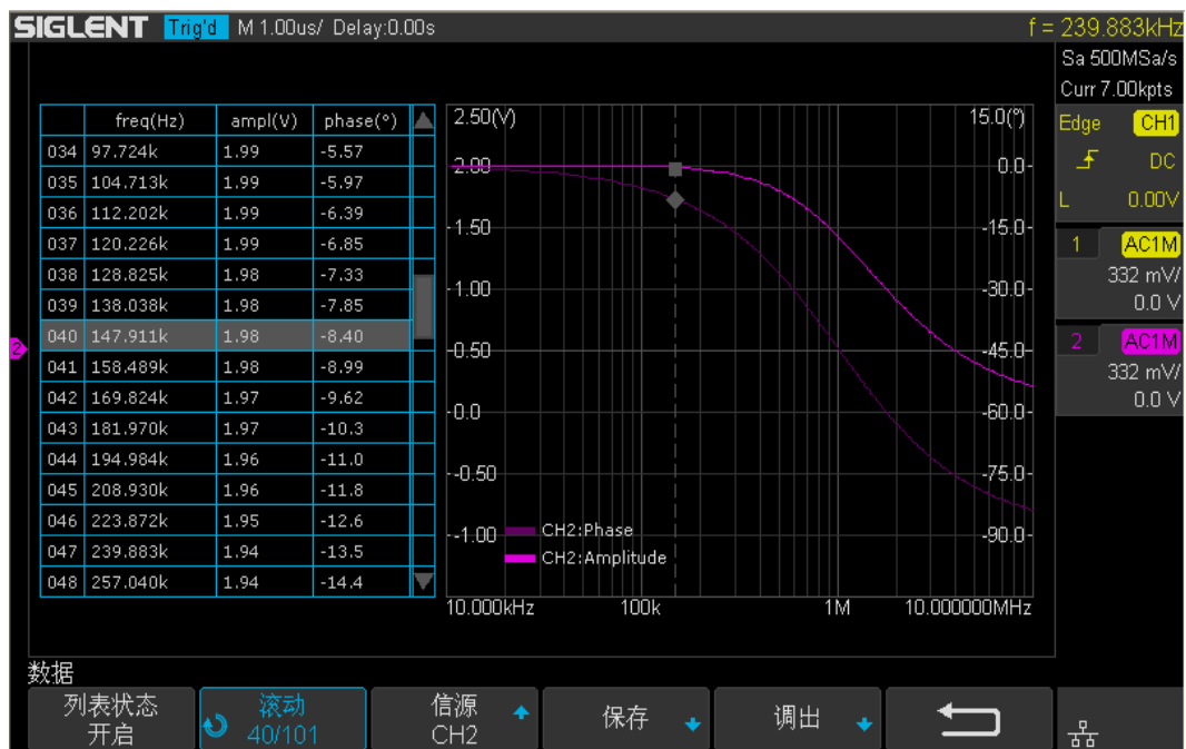
图 163 波特图列表
