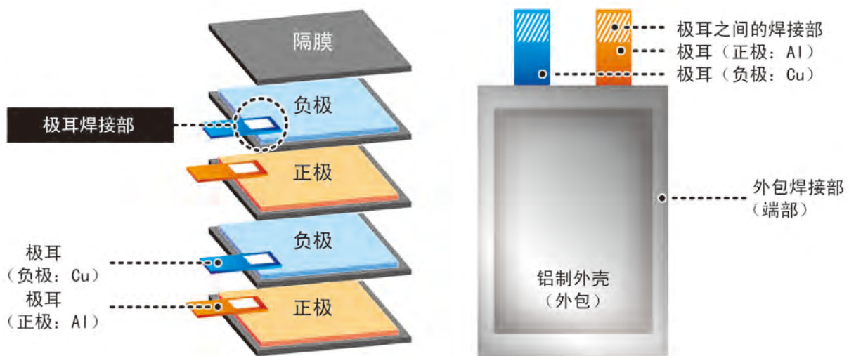
图 8 层叠型锂离子电池的极耳
