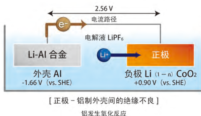
图 19 由于正极-铝制外壳间绝缘不良引起的反应
