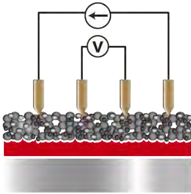
图 5 4 探针测试法
