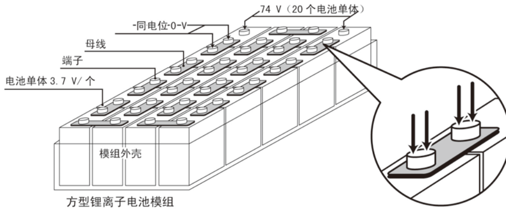
图 42 方型锂离子电池模组的母线连接部电阻测量
