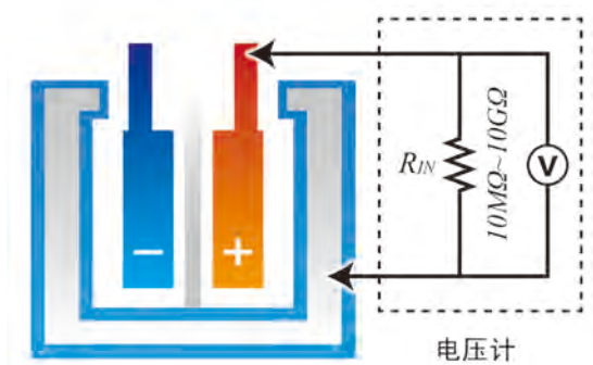
图 20 电压计连接输入电阻 ( R_{IN} ) 的状态
