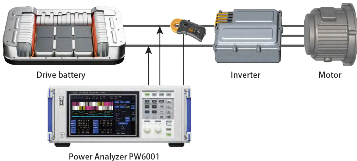
图 47 EV 用变频电机的功率测量
