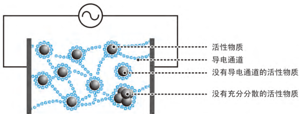
图 3 电极涂层的阻抗测量
