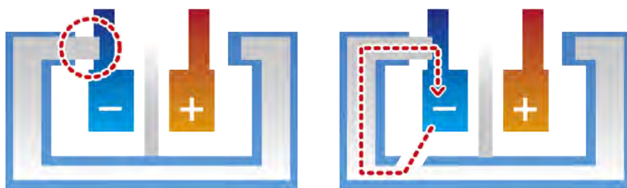
图 17 由于负极绝缘不良与外壳内部产生裂缝形成的电流回路
