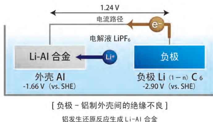
图 18 由于负极-铝制外壳间绝缘不良引起的反应
