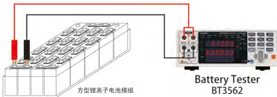
图 41 能安全的进行电阻测量的电池测试仪 BT3562 系列
