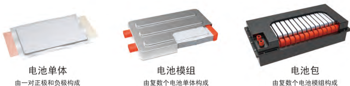
图 39 层叠型锂离子电池的形态示例
