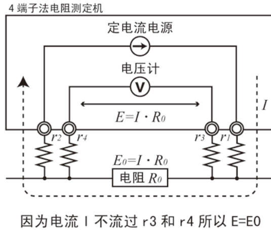
图 10 4 端子法电阻测量
