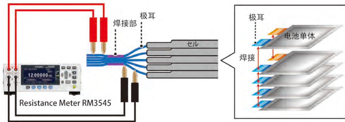
图 40 复数电池单体的极耳焊接部电阻测量
