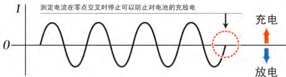
图 33 测量信号的零位交叉停止功能
