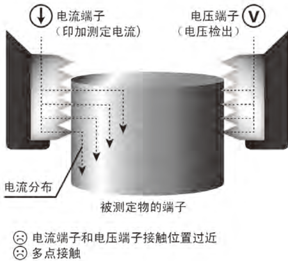
图 34 多点接触的影响
