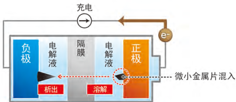
图 23 随着树状晶体的成长将会刺破隔膜
