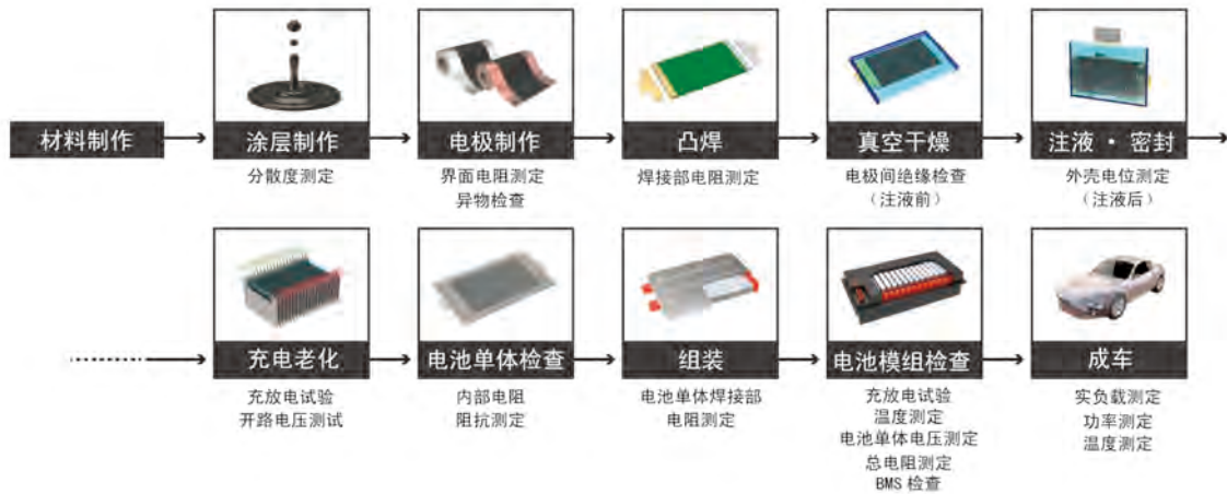
图 1 各工艺检查项目
