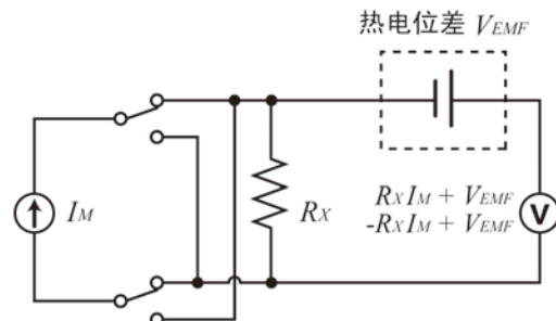
图 12 通过电流反转法消除温差电动势差
