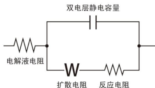
图 28 电池的等价回路示例
