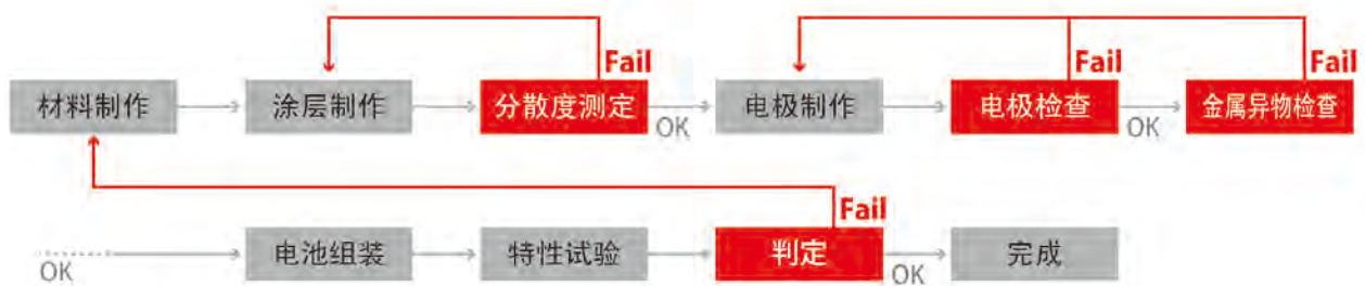
图 2 电池组装工艺的检查
