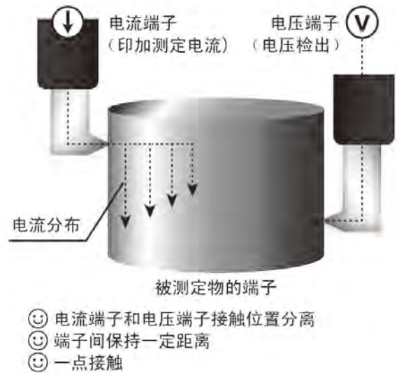
图 35 再现性良好的接触方法
