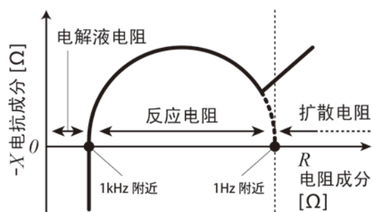
图 27 锂离子电池的科尔图示例
