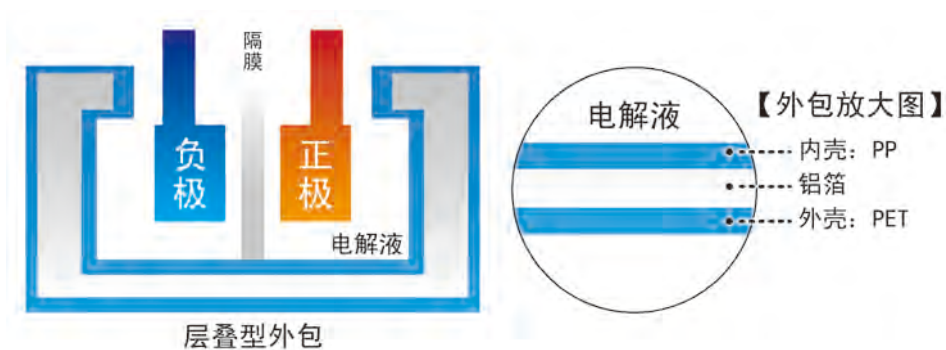
图 16 层叠型锂离子电池的构造图例
