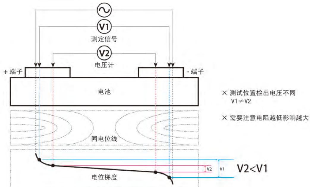
图 36 电流端子和电压端子接触位置的影响
