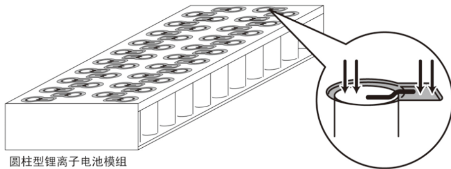
图 43 圆柱型锂离子电池模组的母线连接部电阻测量
