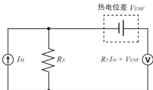
图 11 由温差电动势差产生的误差
