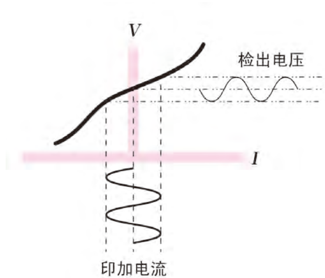
图 32 测量电流合适的情况下的检出电压
