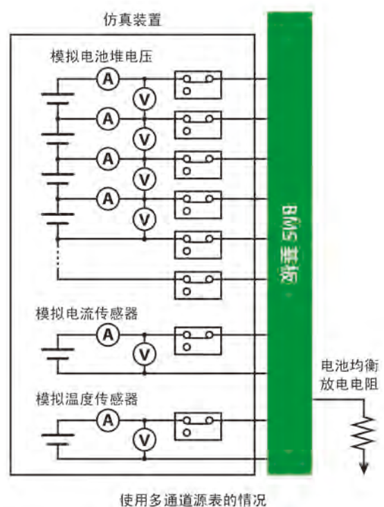
图 45 仿真设备构成示例
