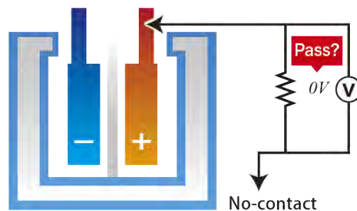
图 21 由于错误接触导致的误判定例
