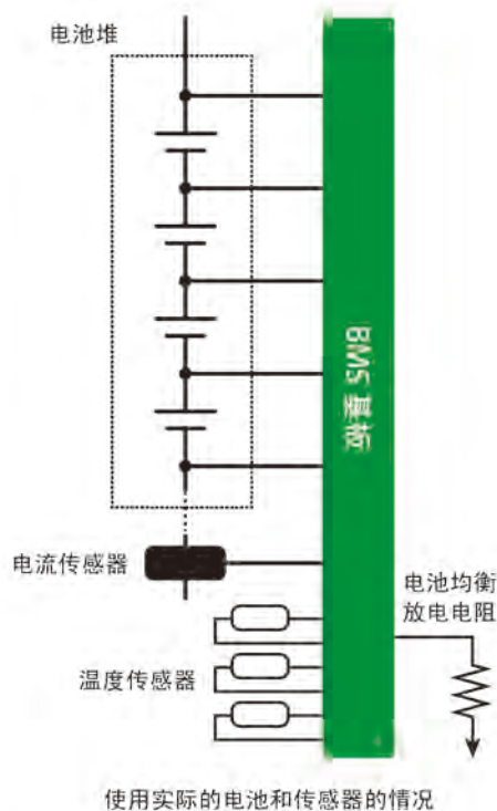
图 44 使用实际电池和传感器的评估设备
