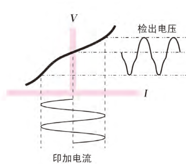
图 31 测量电流过大的情况下检出电压失真
