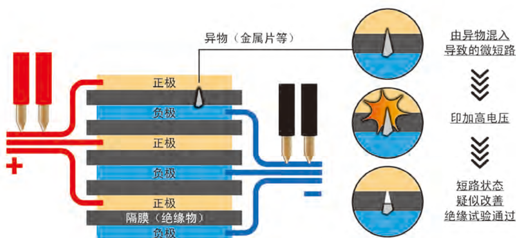
图 15 由于施加高电压导致暂时的微短路改善
