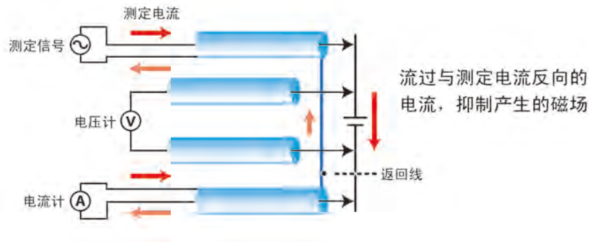
图 30 4 端子对法
