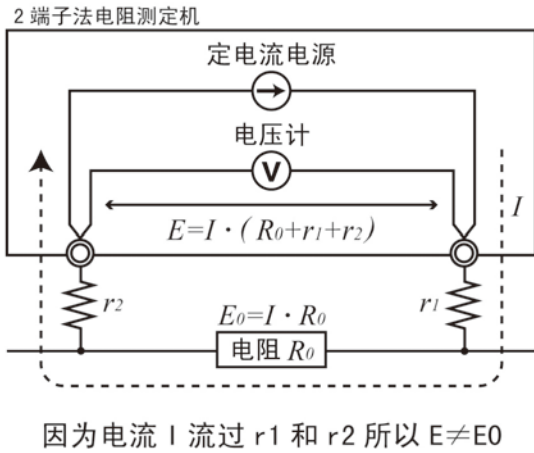
图 9 2 端子法电阻测量
