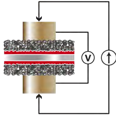
图 6 贯通电阻测试
