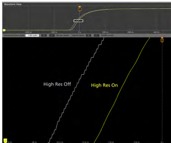
MSO 5B 系列的 12 位 ADC 及新型高分辨率模式实现了业界领先的垂直分辨率。
