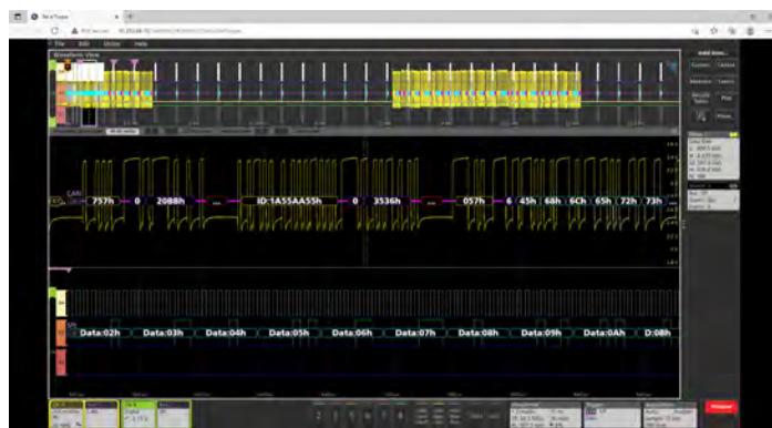
e*Scope 可以使用常用网络浏览器，简便地实现远程查看和控制功能。
