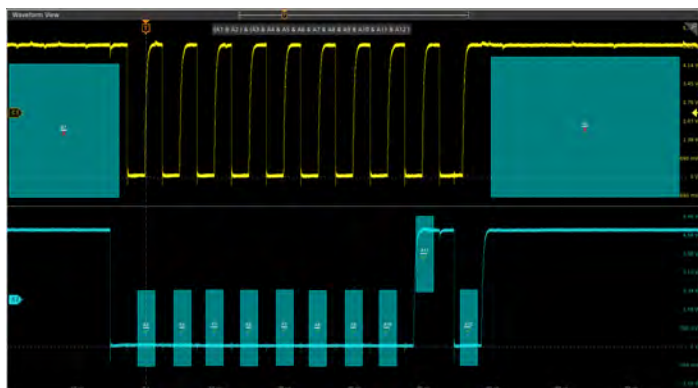
多条通道触发。可视触发区域可以与覆盖多条通道的事件相关，比如在通道1上触发某个突发宽度，在通道2上触发指定的码型。
