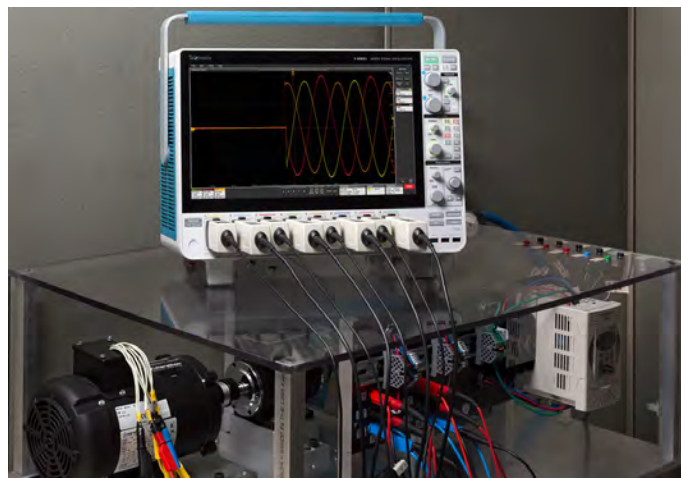
三相马达上的电压测量, 显示了启动后的三相输入电压。
