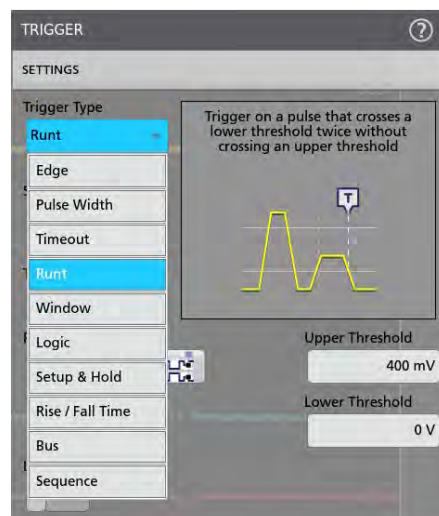
触发菜单中的各种触发类型和上下文相关帮助可以更简便地隔离对应的事件。
