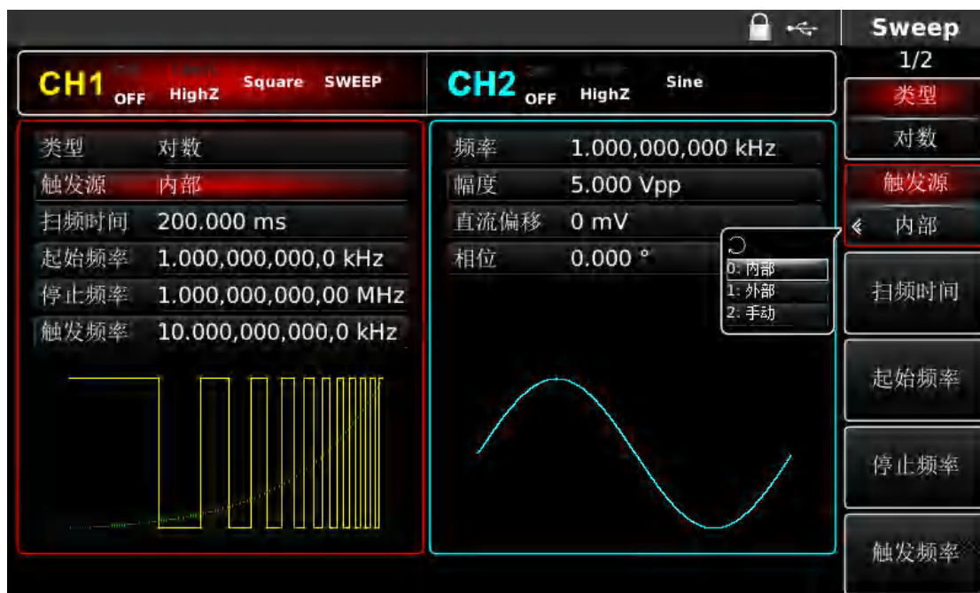
图 4-126 选择触发源
