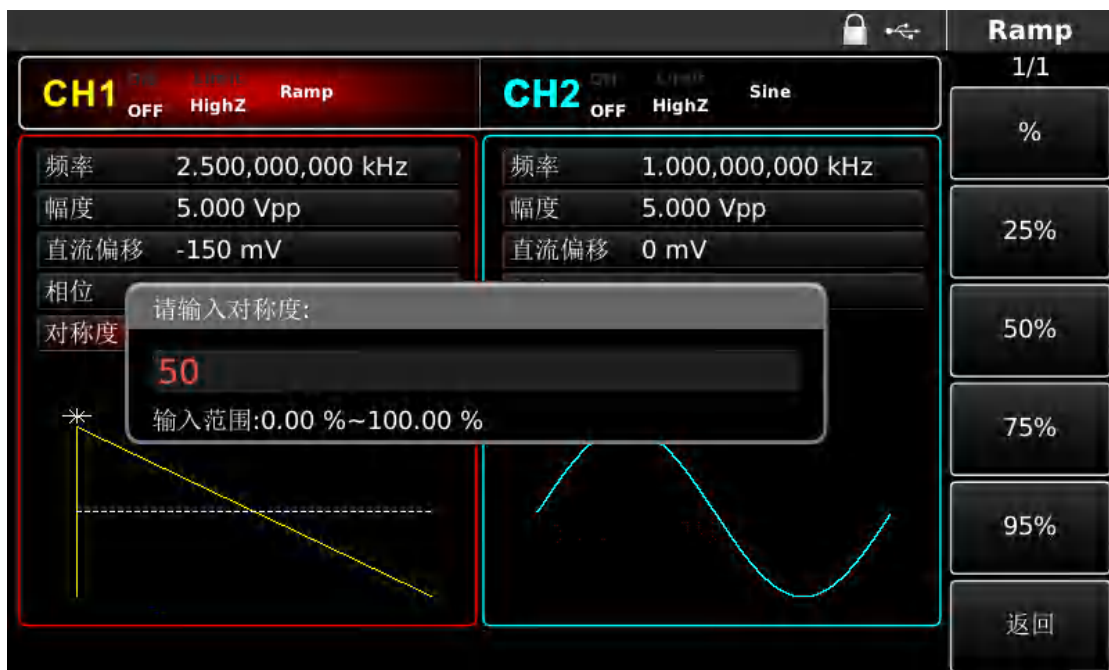
图 3-8 设置对称度
