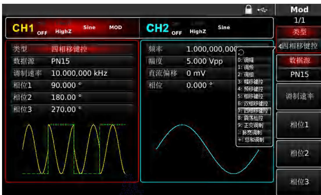
图 4-78 设置四相移键控参数
