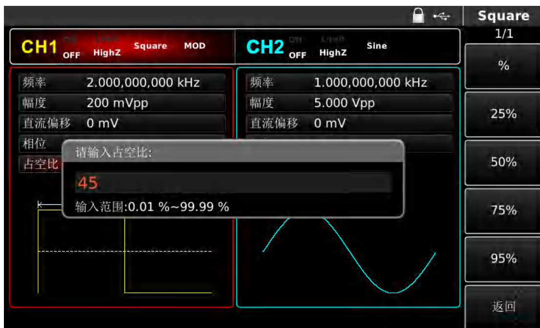
图 4-105 设置载波占空比
