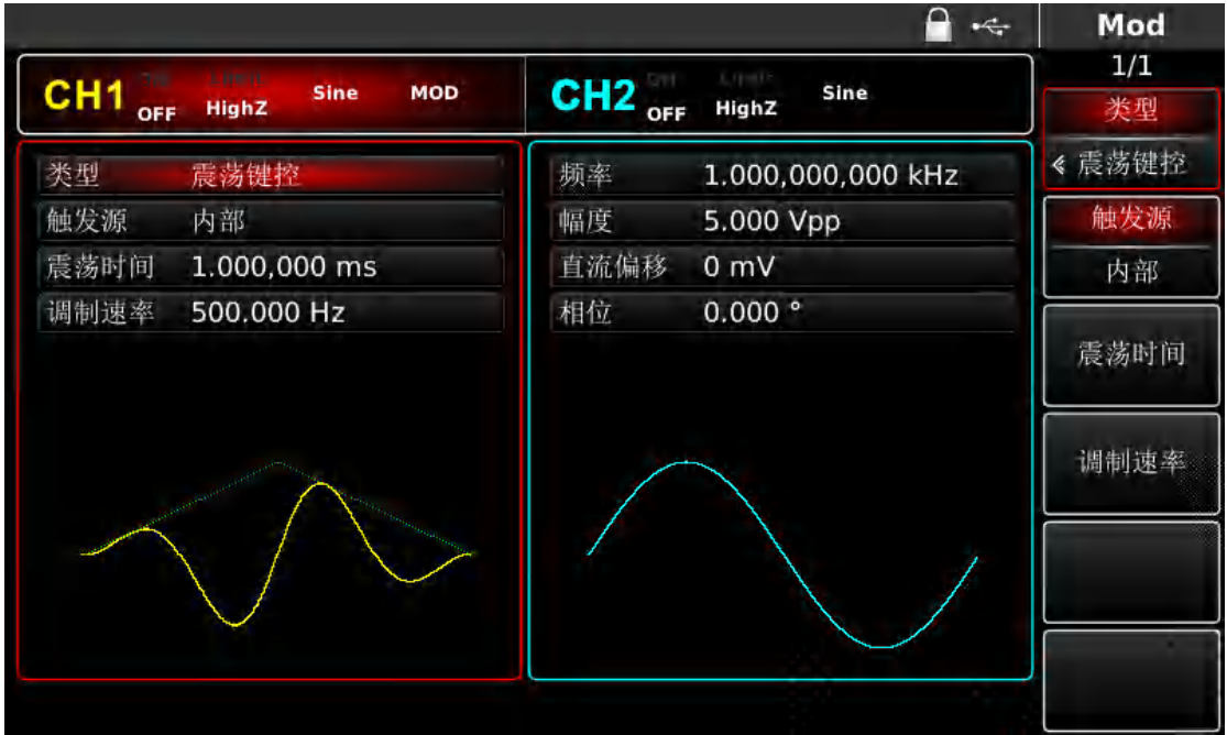
图 4- 84 选择调制源
