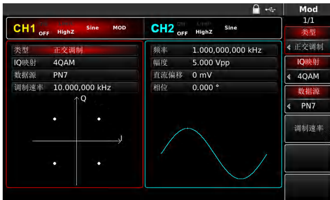
图 4-94 选中正交调制功能
