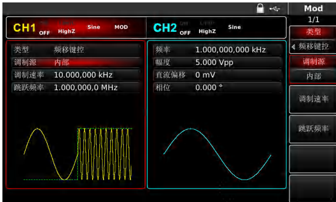
图 4-49 选中调制源
