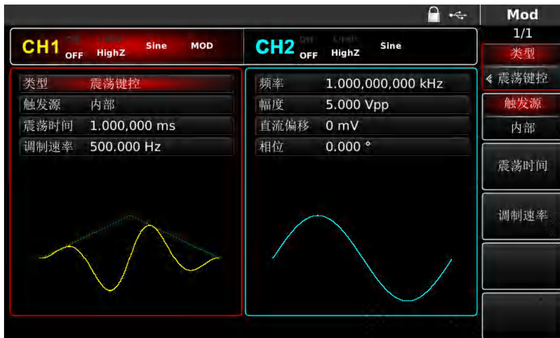
图 4-85 选择调制源
