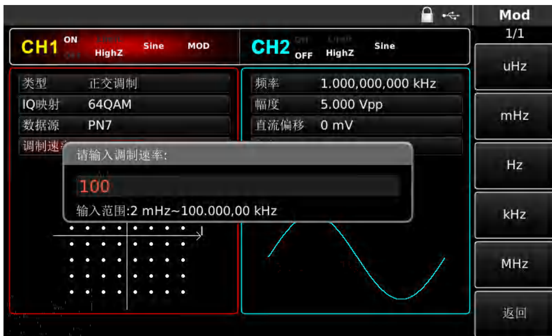
图 4-97 设置调制速率
