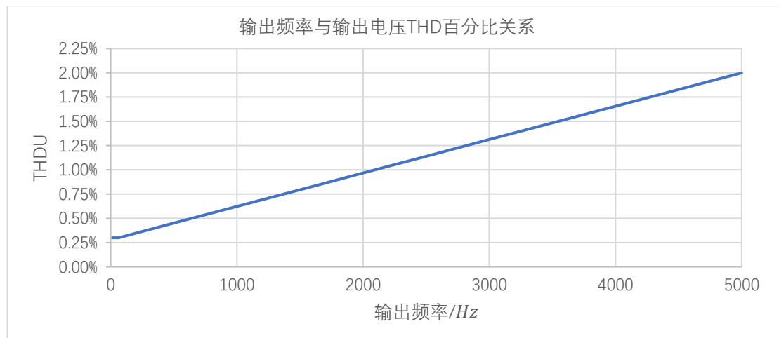
图 10 输出频率与输出电压 THD 百分比关系
