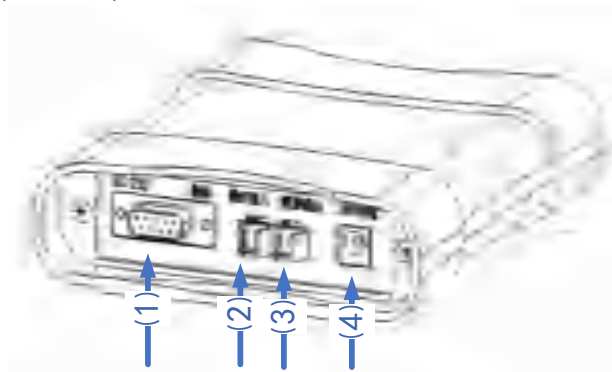
图 95 触发终端后面板功能划分
