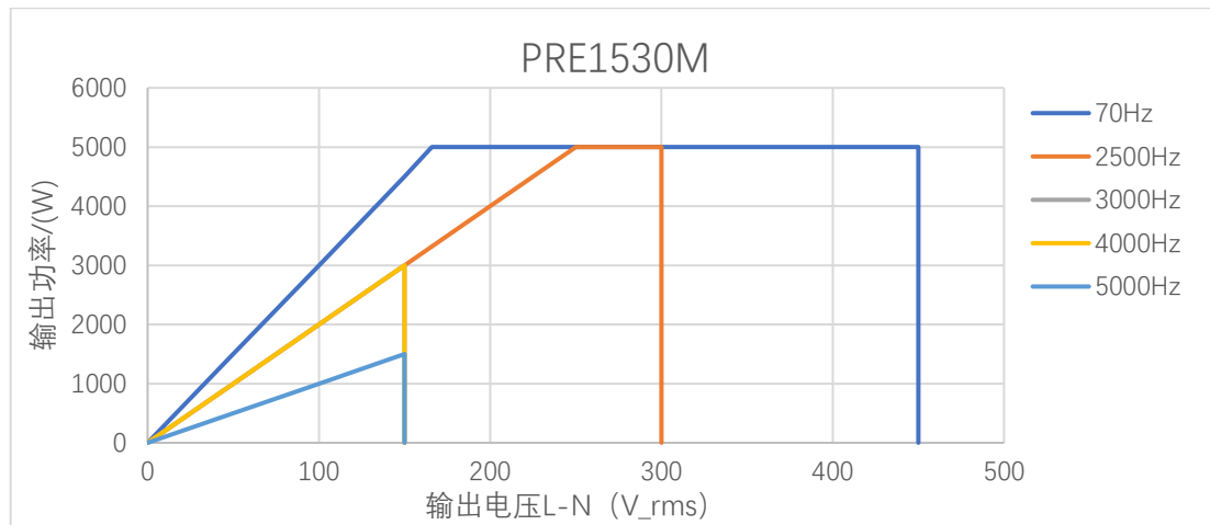
图 9 PRE1530M 三相模式下单相输出电压与输出功率的关系
