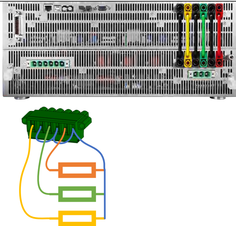
图 26 Y 形负载连接示意图
