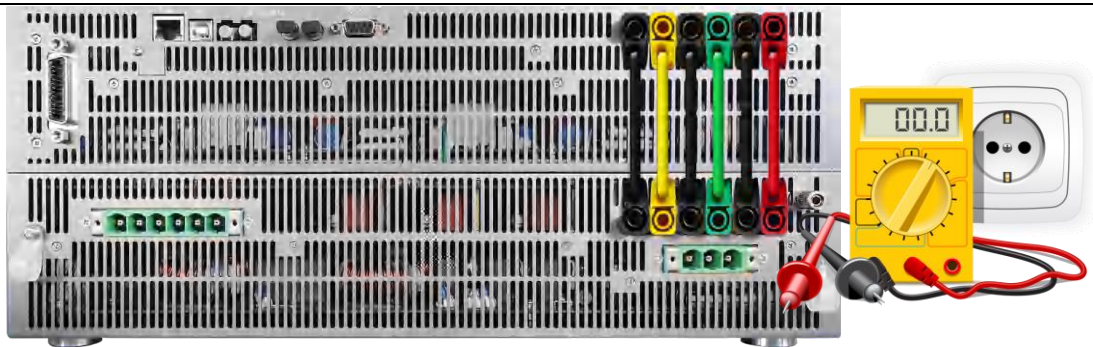
图 1 断开交流电源后的交流输入滤波器剩余电压检查示意图
