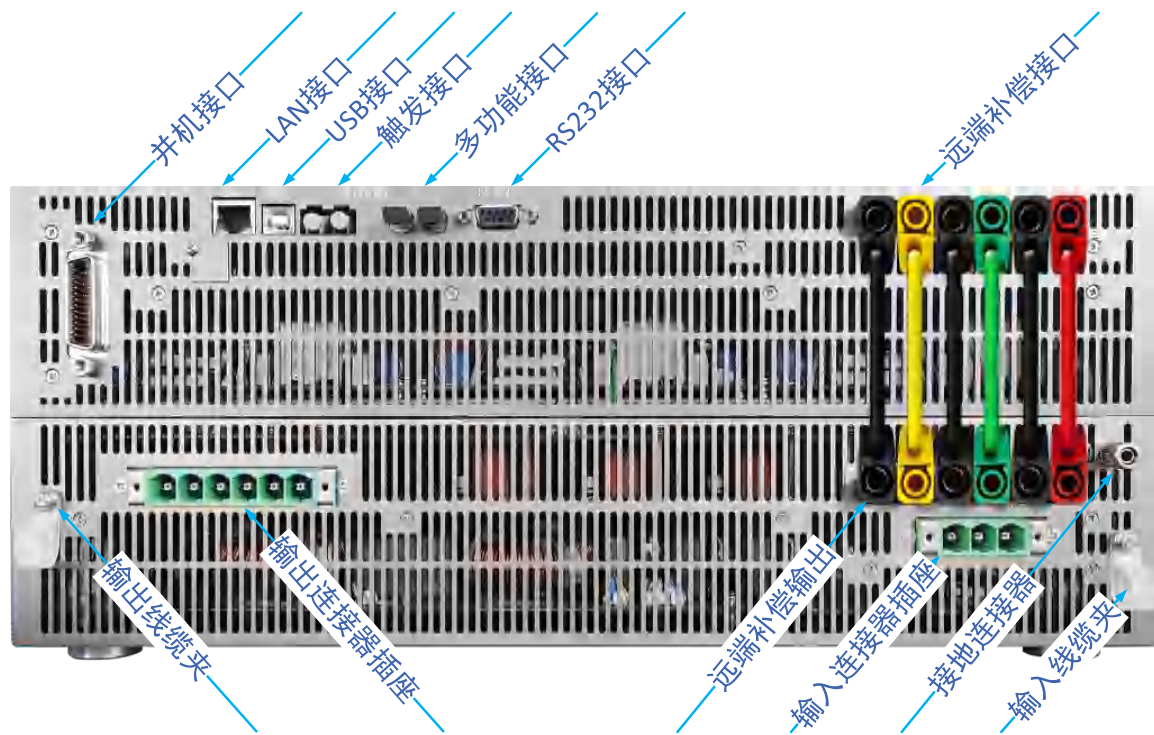
图 23 后面板接口说明图
