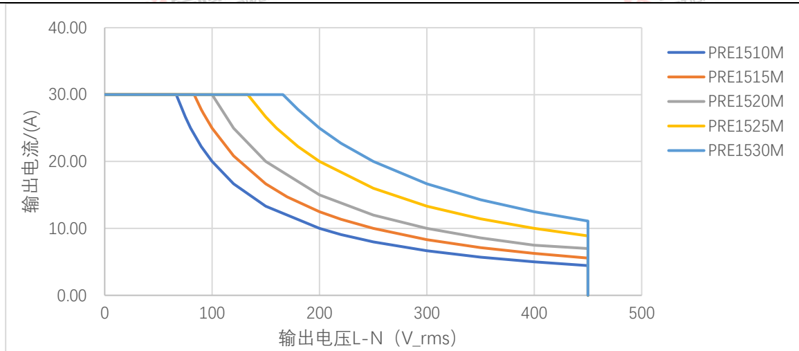
图 4 恒功率曲线图
