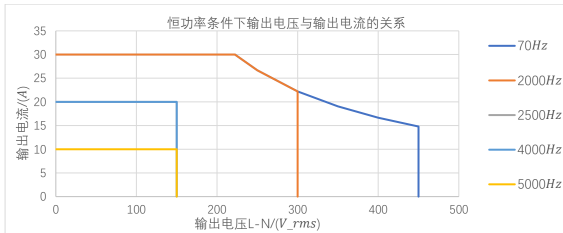
图 11 PRE1530M 在恒功率条件下输出电压与输出电流的关系
