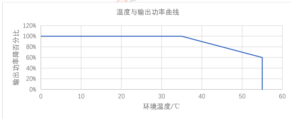
图 19 温度与输出功率曲线
