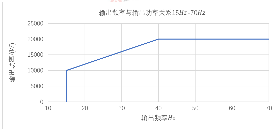
图 12 输出频率与输出功率关系 15Hz-70Hz
