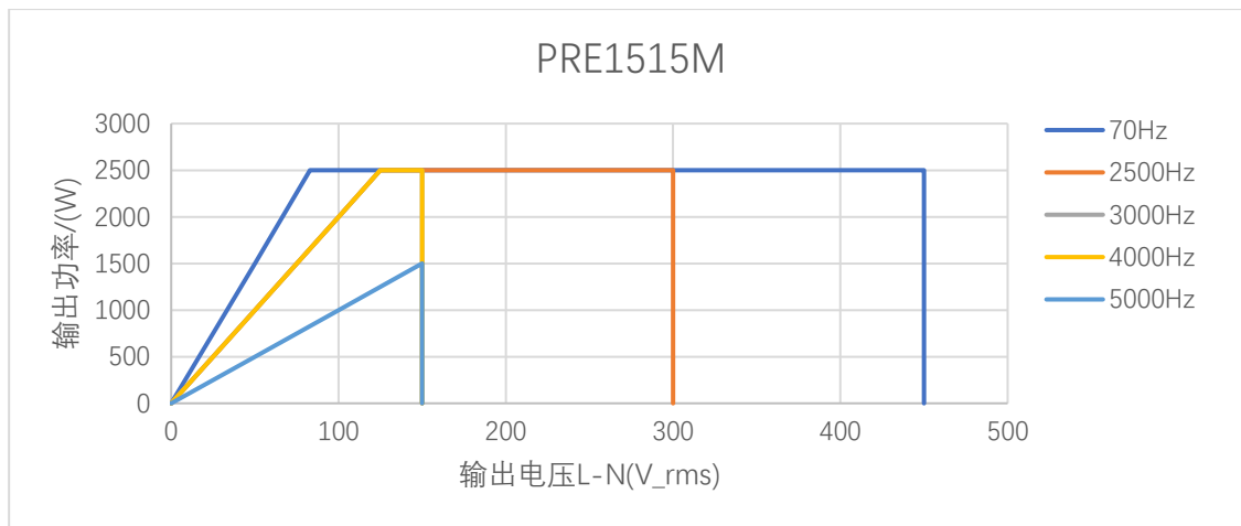
图 6 PRE1515M 三相模式下单相输出电压与输出功率的关系
