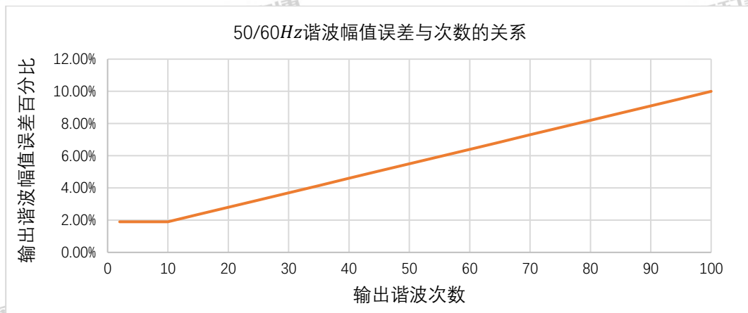
图 14 50/60Hz谐波幅值误差与次数的关系
