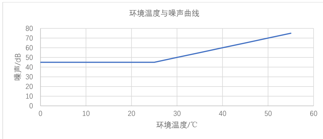
图 20 环境温度与噪声曲线
