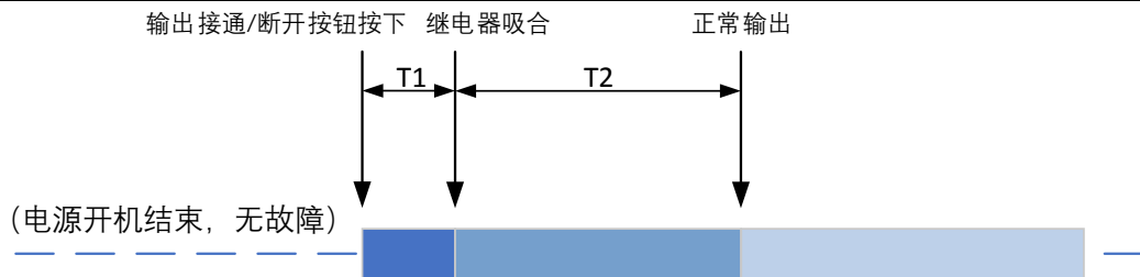
图 41 电源输出时序图
