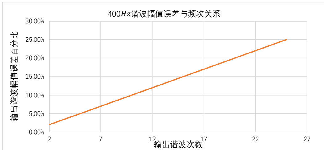
图 15 400Hz谐波幅值误差与频次关系
