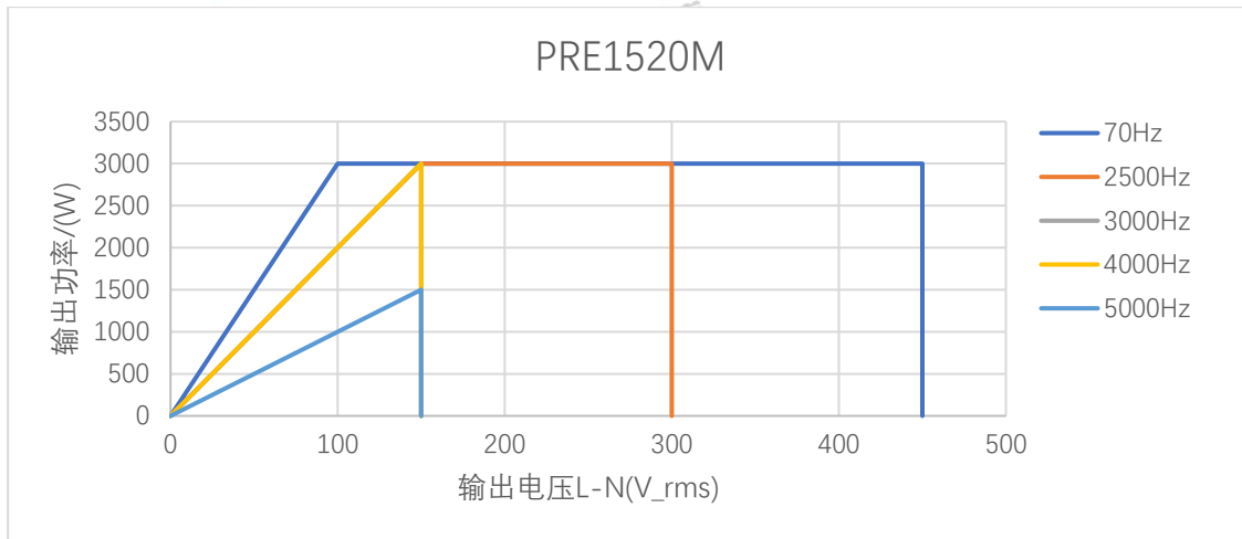
图 7 PRE1520M 三相模式下单相输出电压与输出功率的关系
