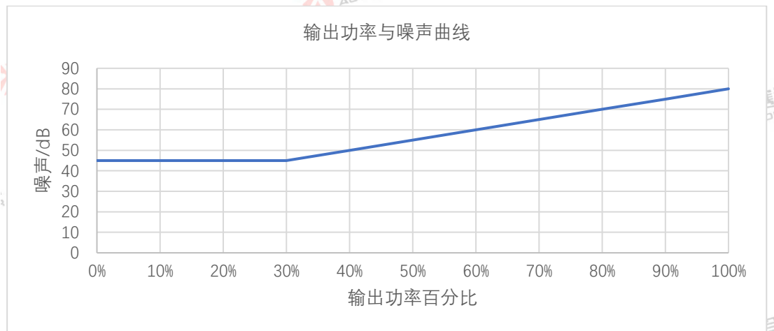
图 21 输出功率与噪声曲线
