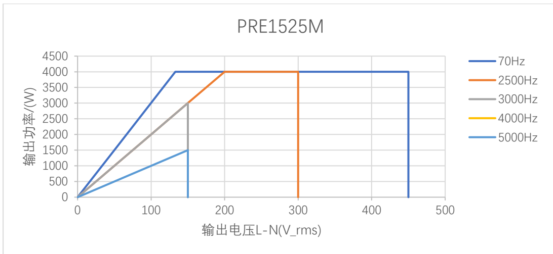
图 8 PRE1525M 三相模式下单相输出电压与输出功率的关系
