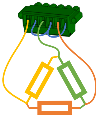
图 27 \Delta 形负载连接示意图
