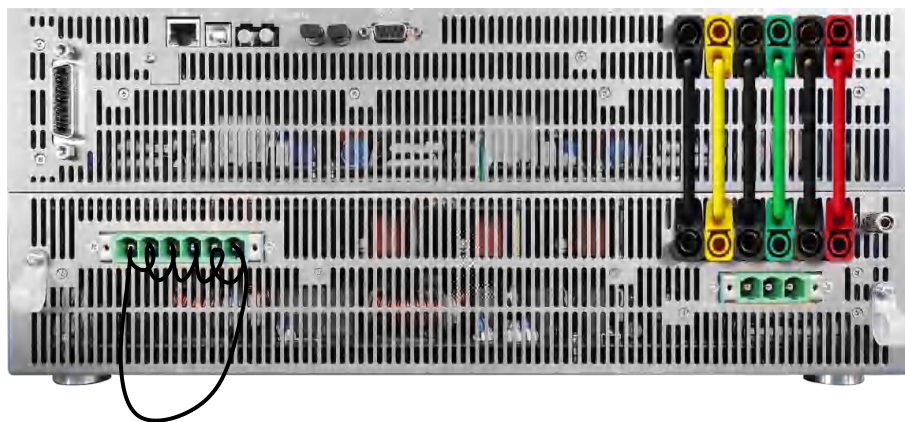
图 65 校准电压零偏接线示意图
