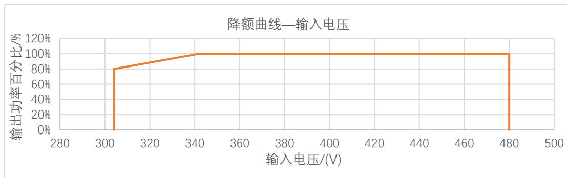
图 17 降额曲线—输入电压
