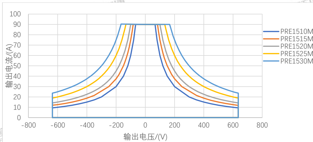
图 16 PRE 系列电源直流恒压模式下输出电压与输出电流关系
