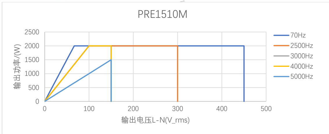
图 5 PRE1510M 三相模式下单相输出电压与输出功率的关系
