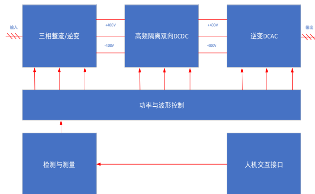
图 2 PRE 系列功能框图
