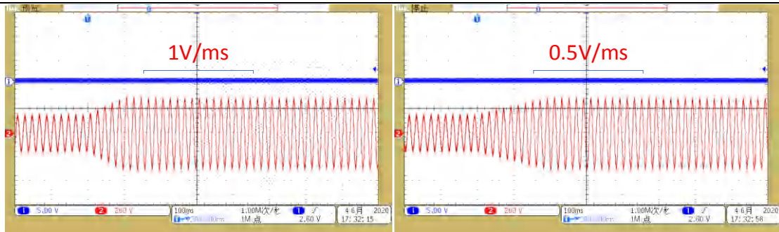
图 56 交流分量斜率示例
