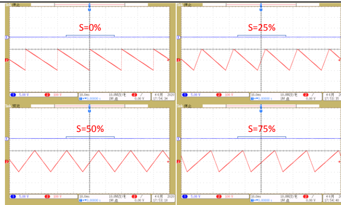
图 55 三角波对称度波形示例
