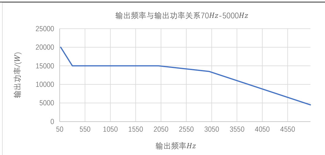
图 13 输出频率与输出功率关系 70Hz-5000Hz
