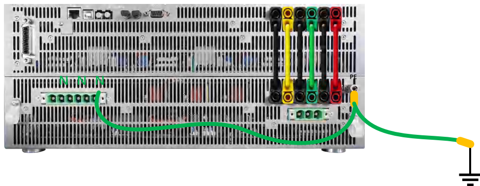
图 24 输出中点接地示意图
