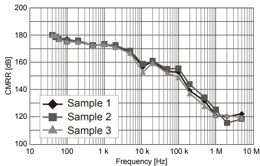
导体位置的影响 (典型值) (100 kHz时)
