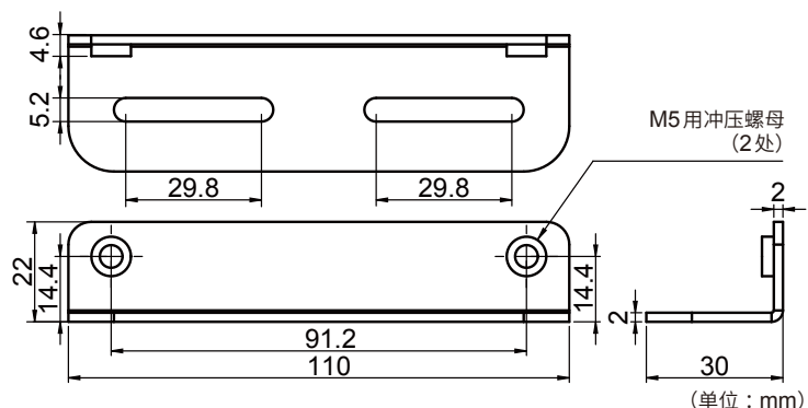
固定配件的尺寸 (选件)
