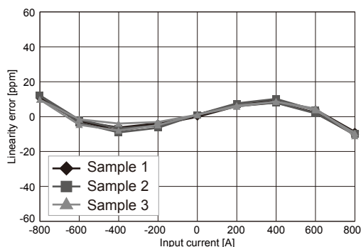
线性误差 (典型值)
