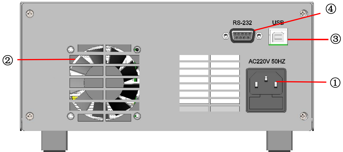
图 2.3.1 设备后面板
