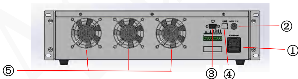
图 2.3.1 负载后面板
