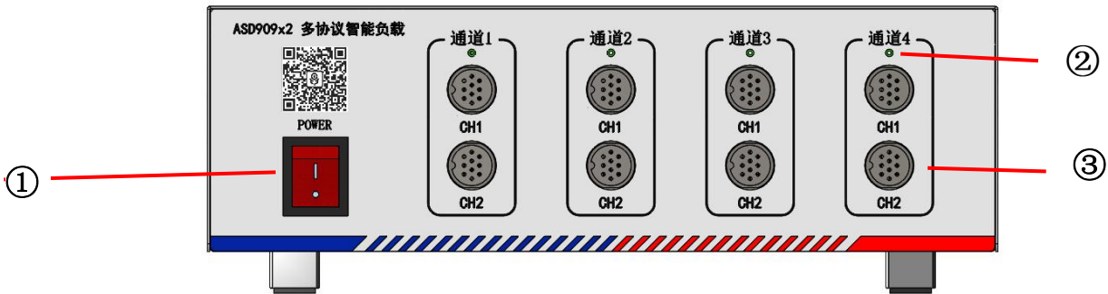
图 2.2.1 主机前面板
