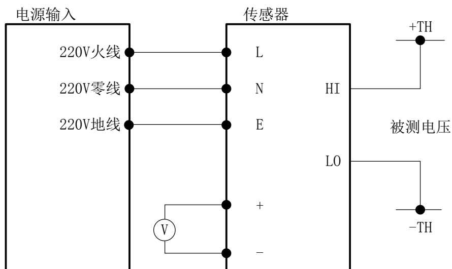
图 2 电气连接图
