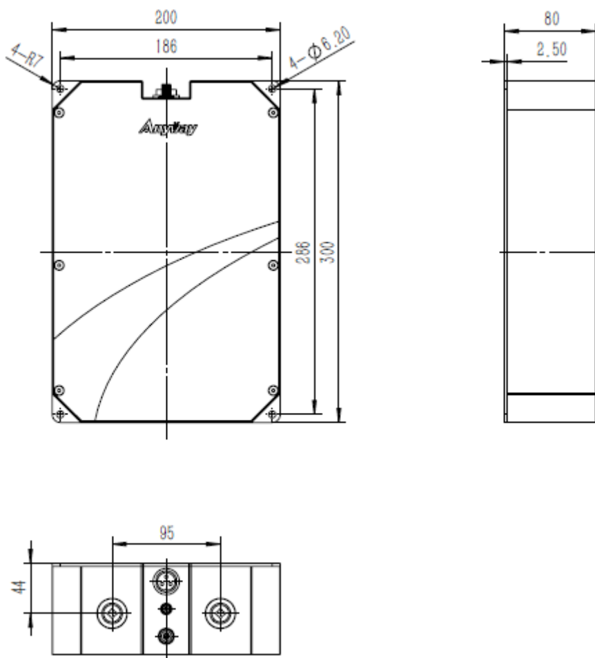
图 1 外形图
