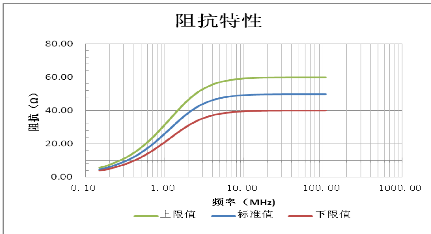
阻抗特性图
