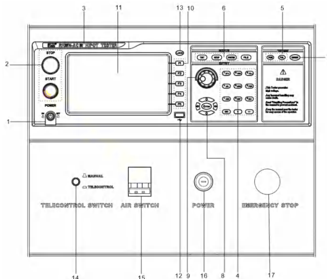
图10 -1前面板说明
