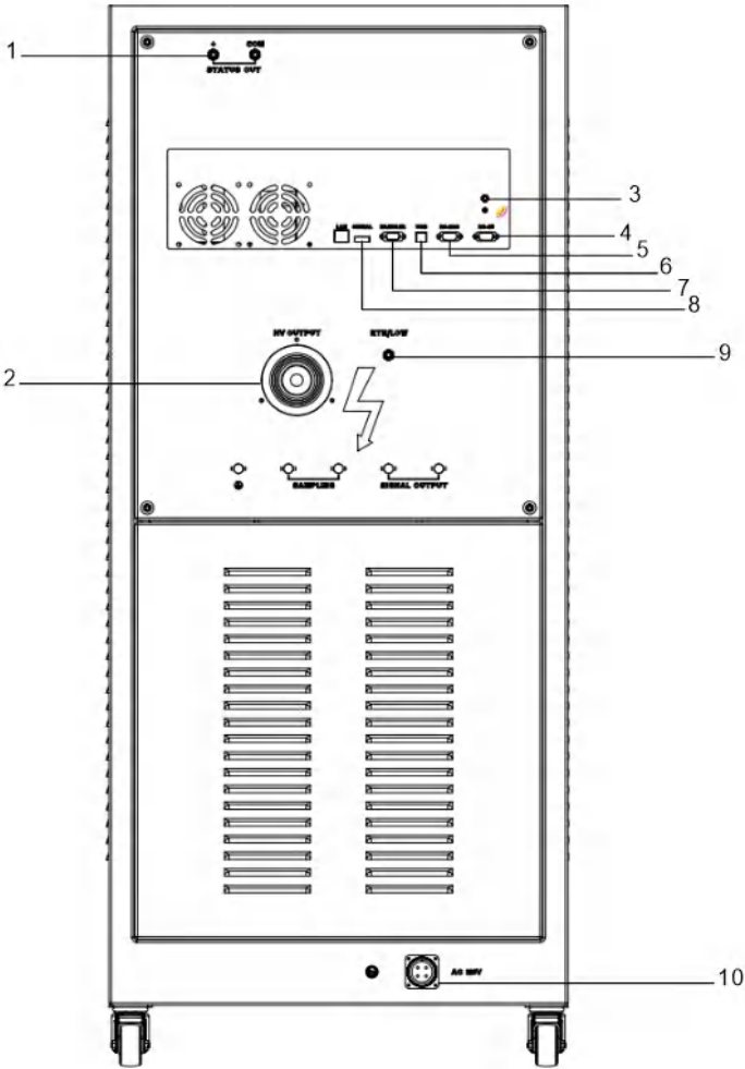
图10-2-1 后面板说明
