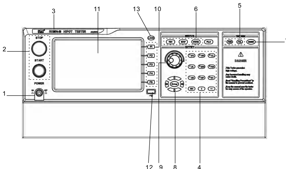
图9-3 前面板
