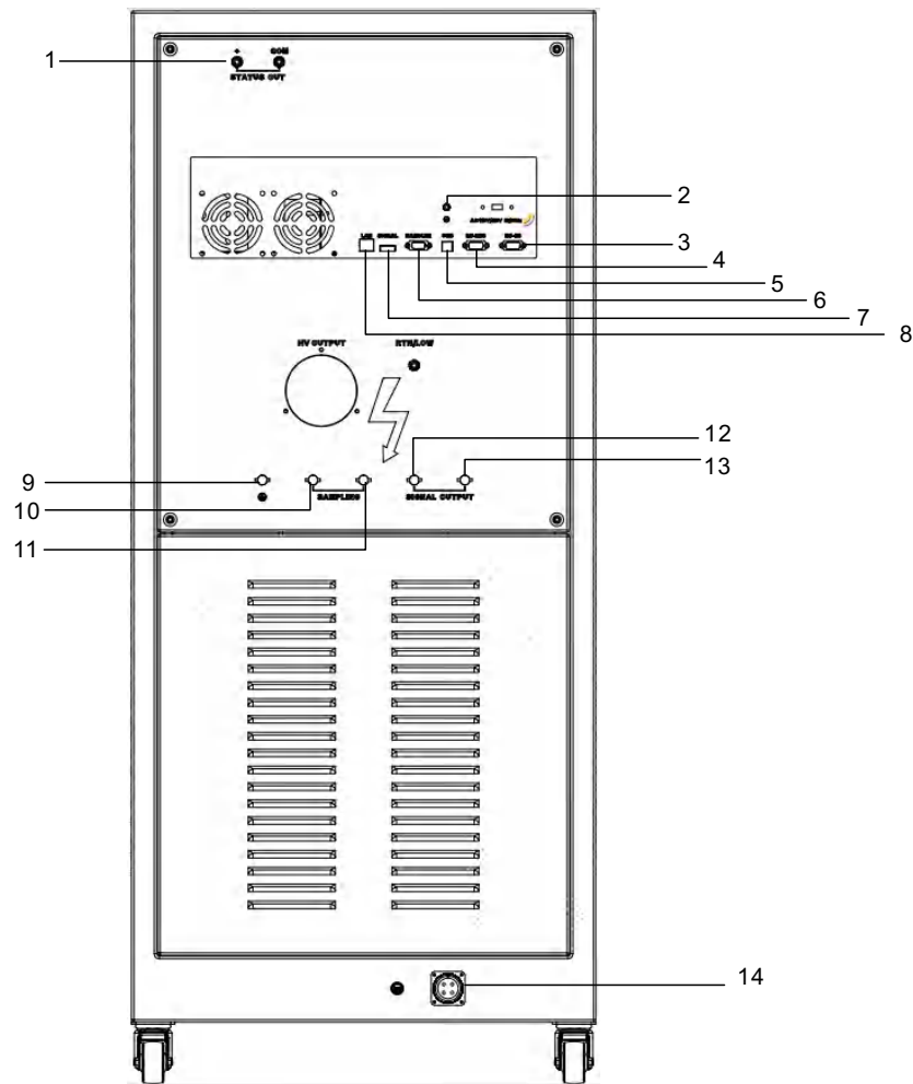
图10-2-2 后面板说明
