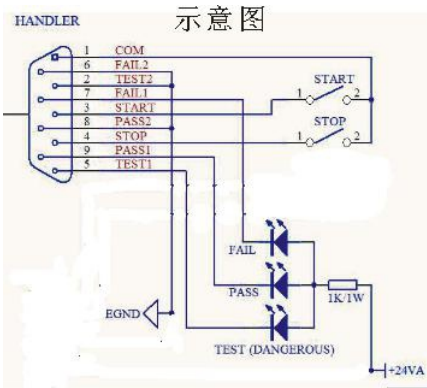
PLC外部接线示意图
