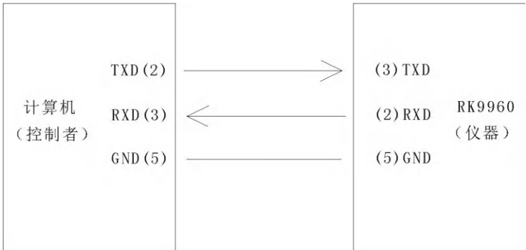
计算机与仪器连接示意图
