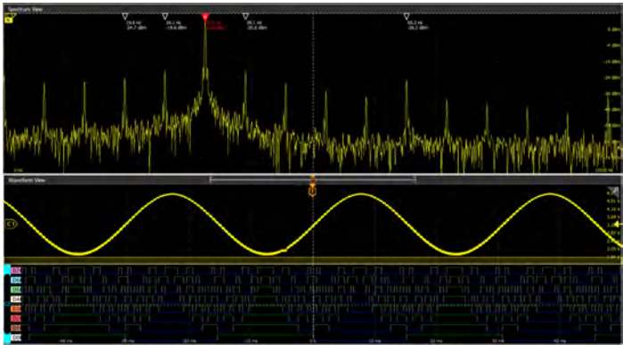
直观的频谱分析仪控制功能如中心频率、频宽和解析带宽(RBW) 独立于时域控制功能，可以简便地进行设置，实现频域分析。每个 FlexChannel 模拟输入有一个频谱视图，可以实现多通道混合域分析。
