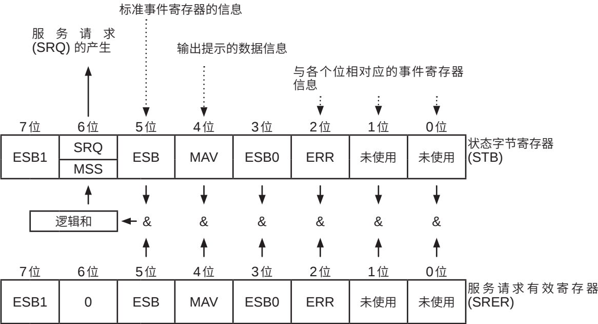
服务请求发生的概念图
