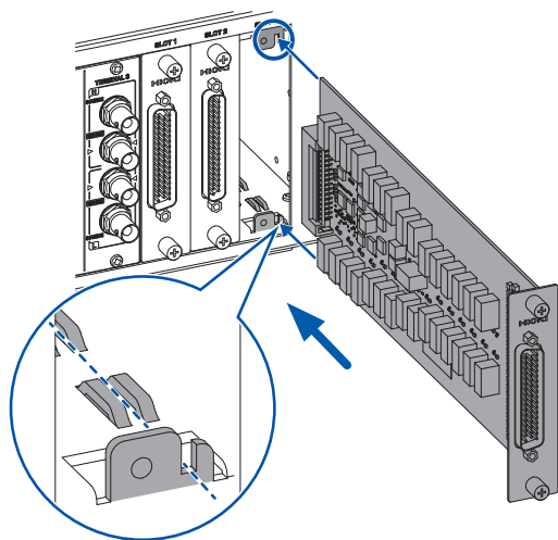
对准导轨
