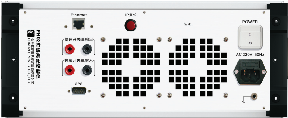
图 2 - 1 - 2 PH02 行波测距校验仪后面板图
