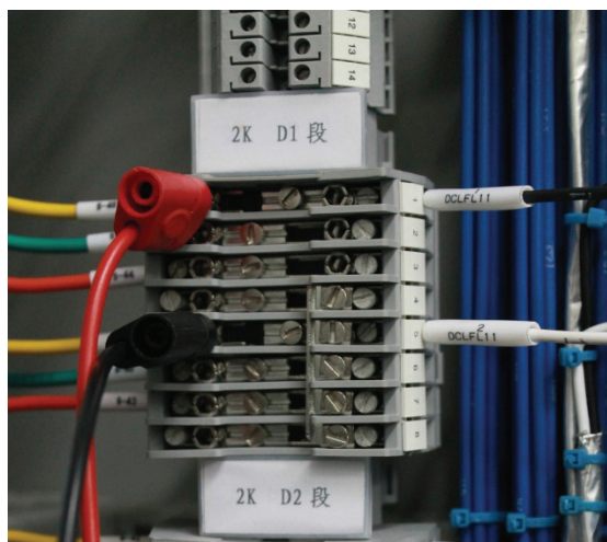
图 4-1-2 测试线连接
