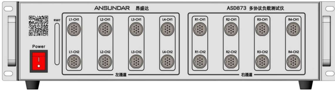
图 2.2.1 负载前面板
