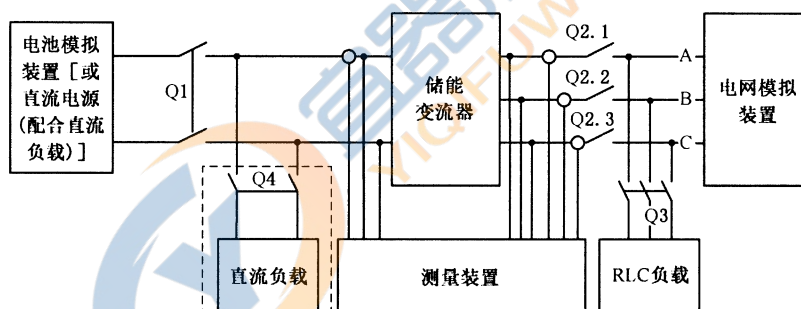
图 2 检测回路示意图
