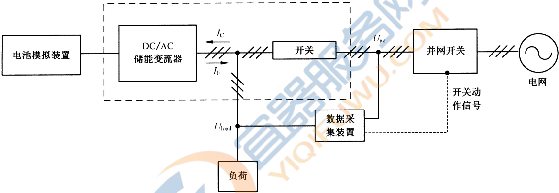
图 3 并离网切换检测回路示意图
