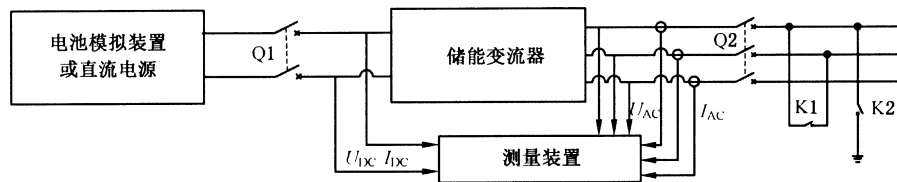
图 12 短路保护检测回路示意图
