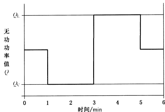
图7 无功功率控制曲线
