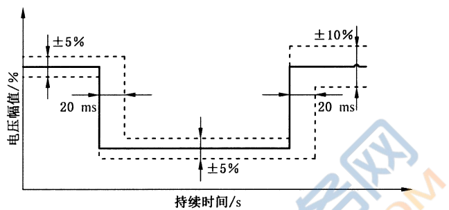
图 10 电压跌落容差
