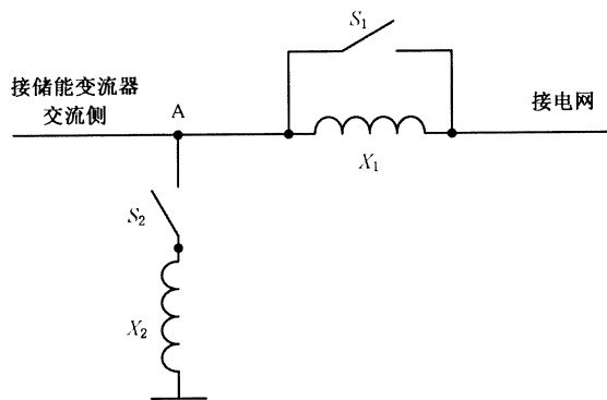
图 1 电压跌落发生装置示意图
