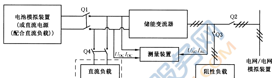
图 4 储能变流器效率检测回路框图
