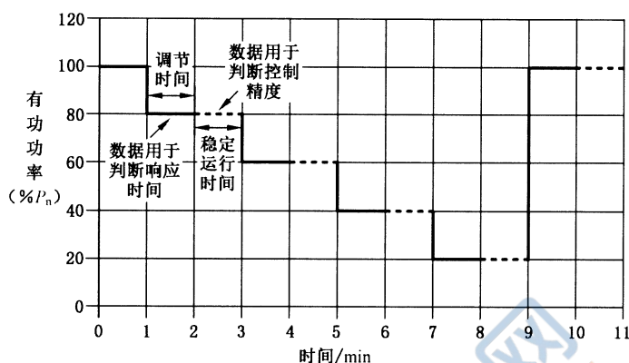
图 6 有功功率控制曲线
