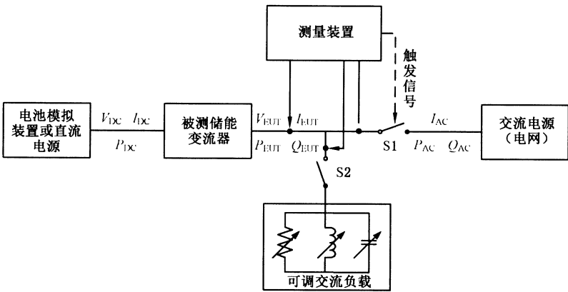
图 11 防孤岛保护检测回路示意图
