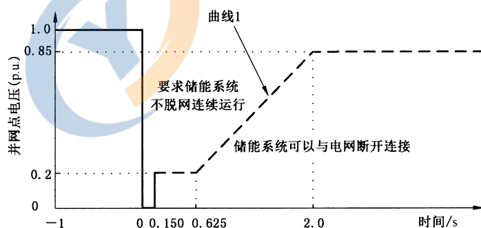
图 9 低电压穿越曲线
