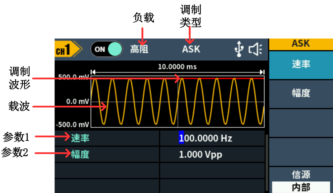
图 5-16 幅移键控调制的用户界面
