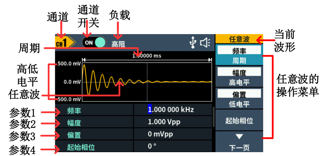
图 5-10: 任意波用户界面
