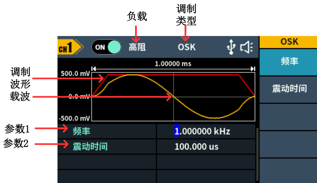
图 5-23 振荡键控调制的用户界面
