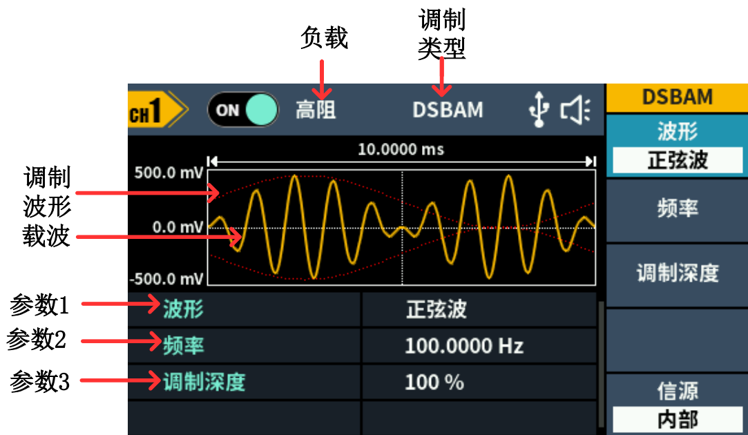
图 5-12：双边振幅调制的用户界面
