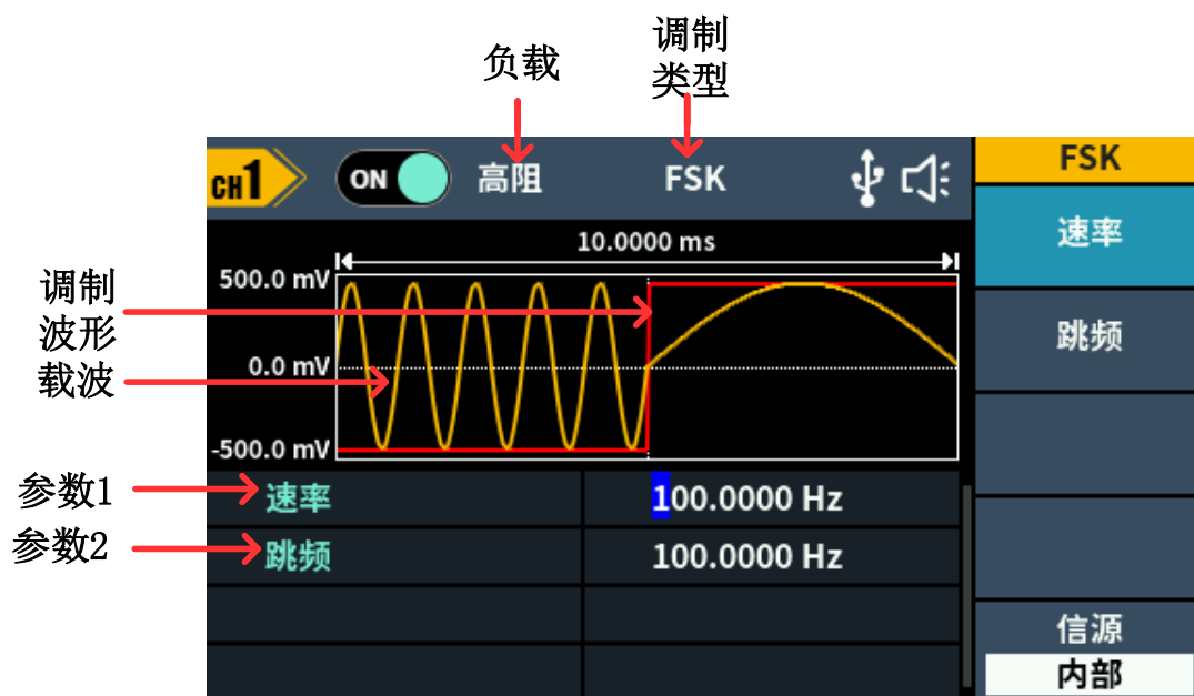
图 5-18：频移键控调制的用户界面
