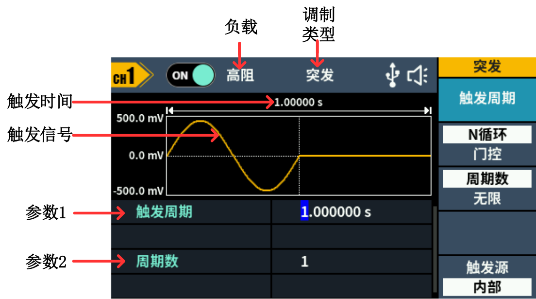
图 5-26：N 循环脉冲串的用户界面
