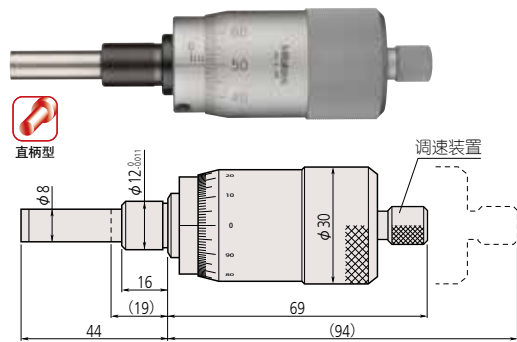
152-102 MHL1-25 质量: 230g
