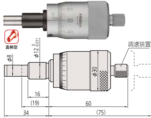
152-101 MHL1-15 质量: 220g
