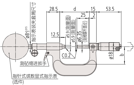
测量范围小于75mm OMD-75R
