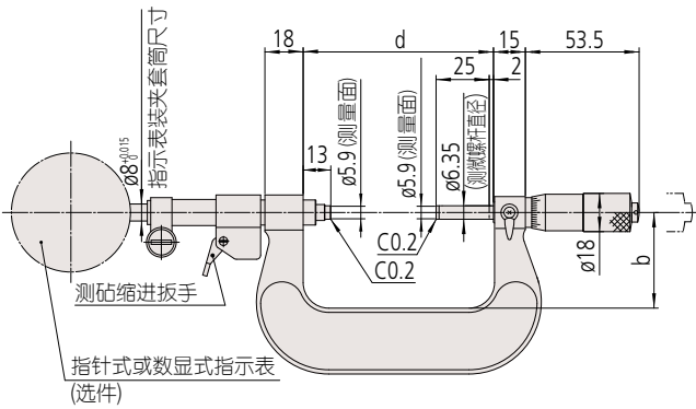
测量范围小于200mm OMD-100R - 200R
