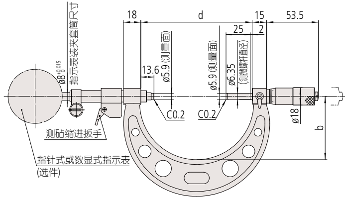
测量范围小于75mm OMD-75R
