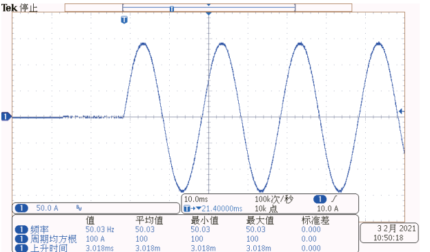
50Hz-100A测试 上升时间为3.1mS
