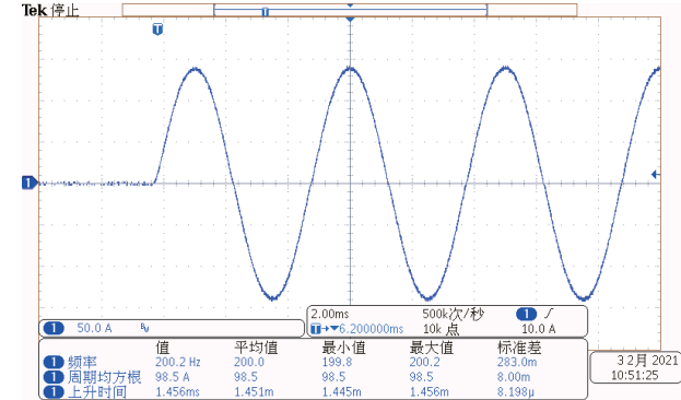
200Hz-100A测试 上升时间为1.5mS
