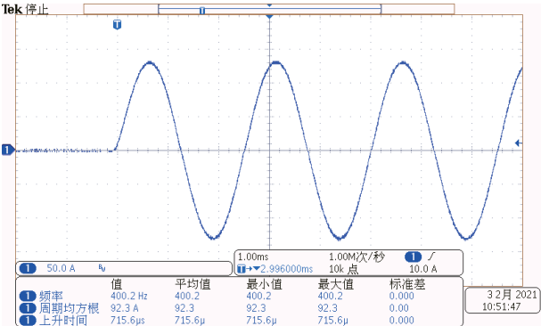
400Hz-100A测试 上升时间为720uS
