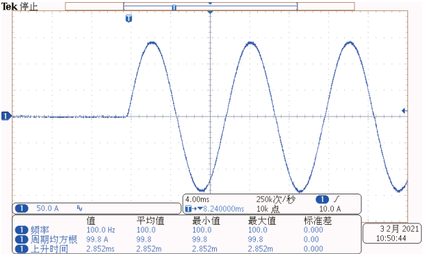
100Hz-100A测试 上升时间为2.9mS
