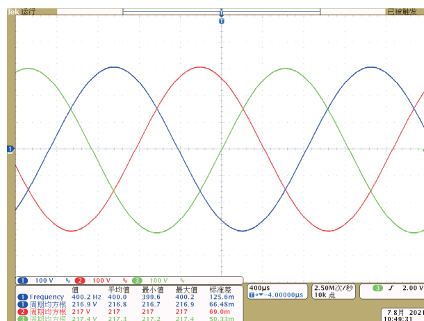
三相相位差120°
