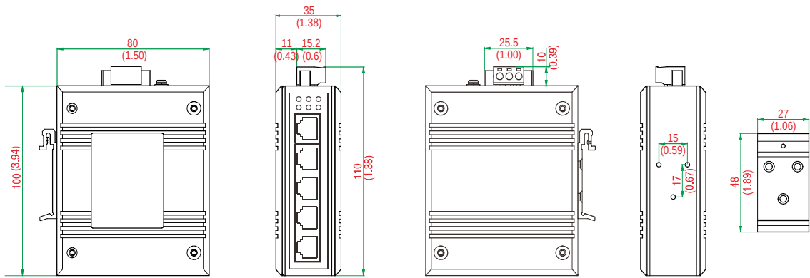
左侧视图
