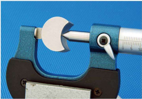
测量异形零件根部尺寸
