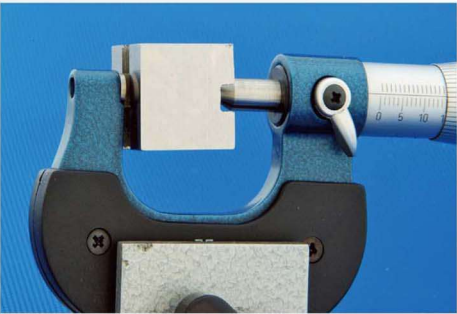
测量槽根部尺寸
