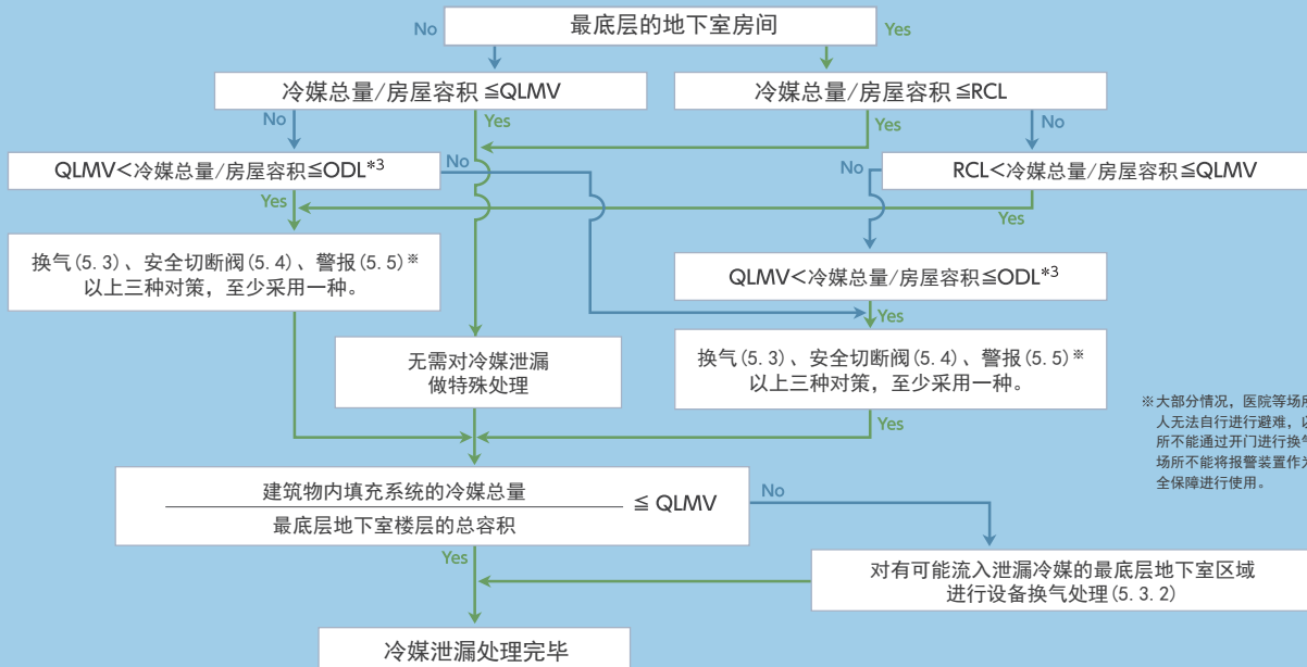
[冷媒泄漏过程图（以JRA GL-13为基础制作）]
