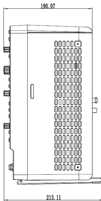
右视图
