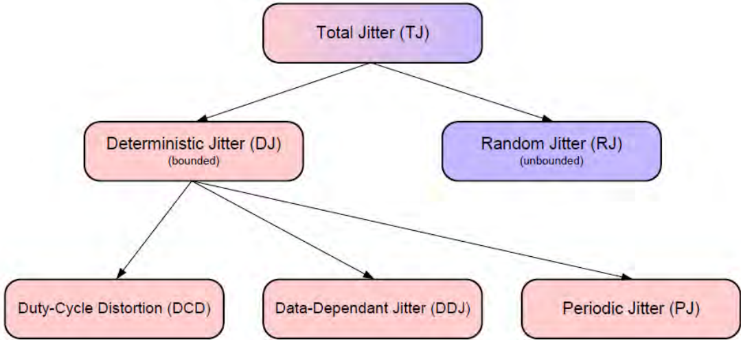
图 33.1 抖动的分解
