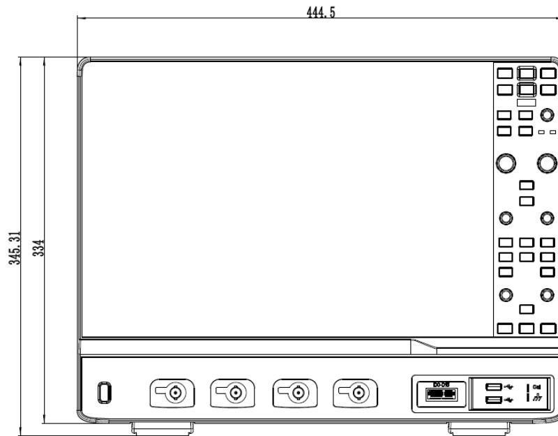
正视图
