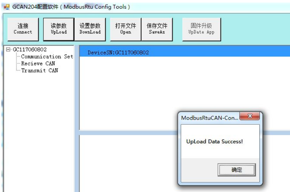
图 4.3 GCAN-204-Config-CH-3.12 软件主界面
