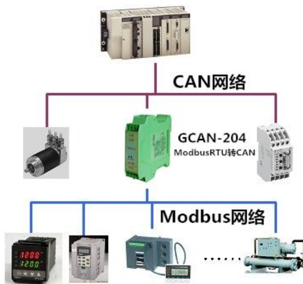
图 2.1 GSCAN-204 模块典型工作环境
