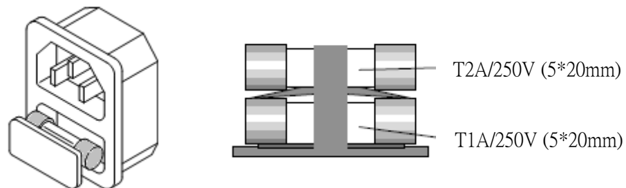
圖 2-2 保險絲座
