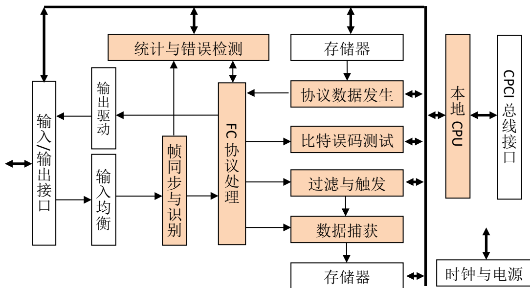
图 3-1 4G FC 总线测试模块原理框图
