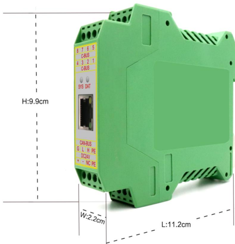
图 2.1 GCAN-301 模块外形尺寸
