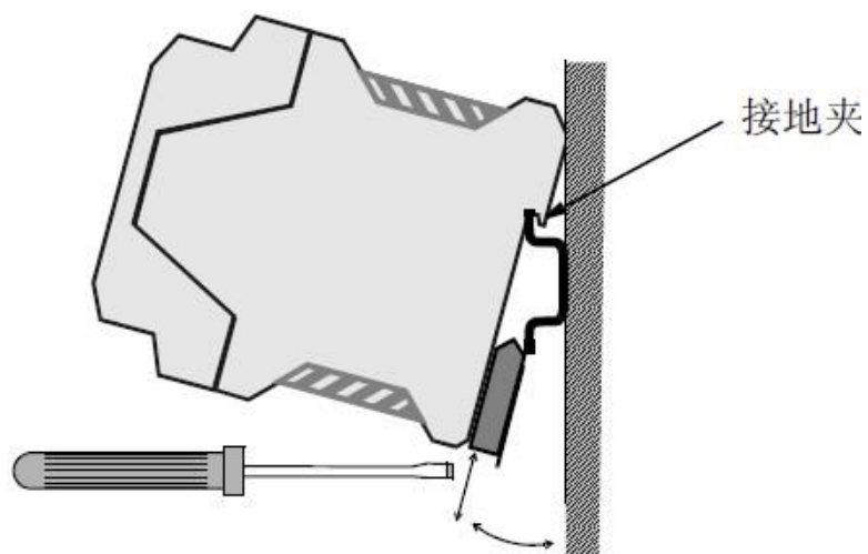
图 2.2 GCAN-302 模块安装
