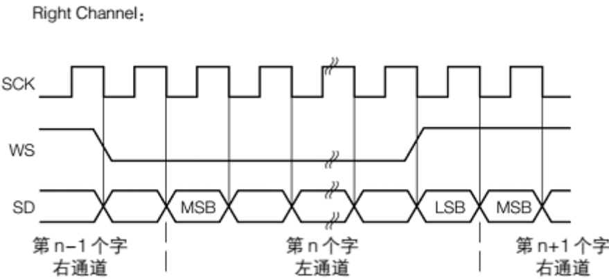
图3.226 I2S 总线时序图
