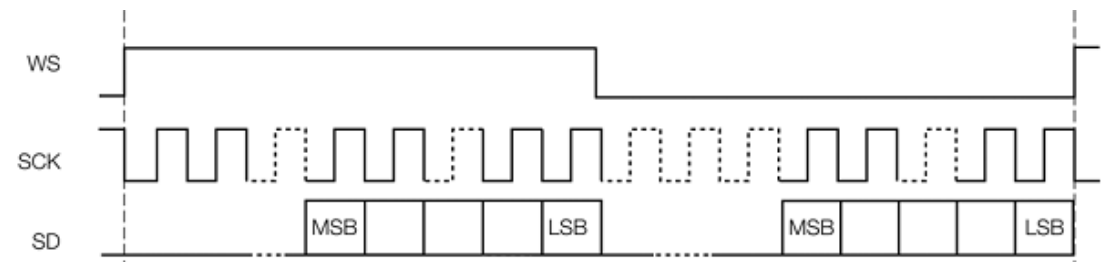
图3.228 RJ 总线时序图
