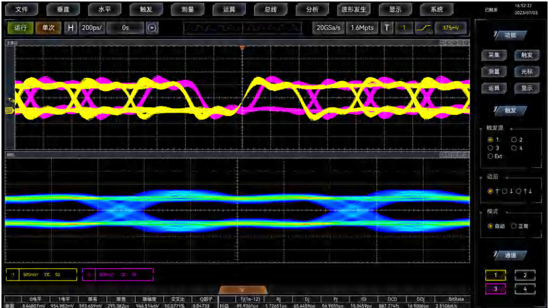
图3.322 眼图示例
