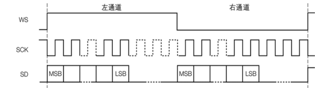
图3.227 LJ 总线时序图
