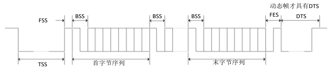
图3.207 FlexRay 帧序列
