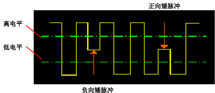
图3.33 窄脉冲脉冲示意图
