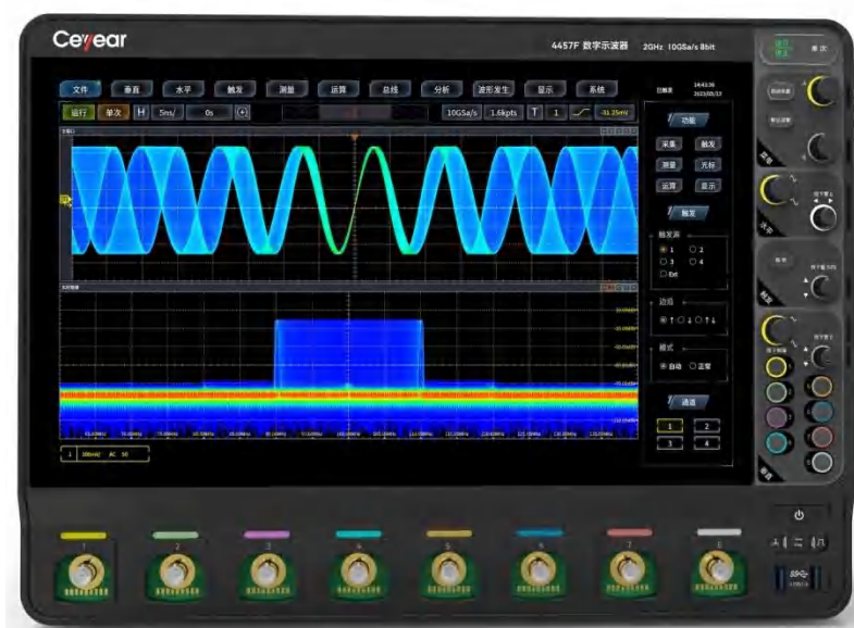
图3.1 前面板
