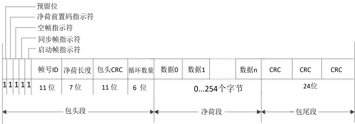
图3.206 FlexRay 帧格式
