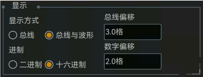
图3.212 FlexRay 显示设置菜单
