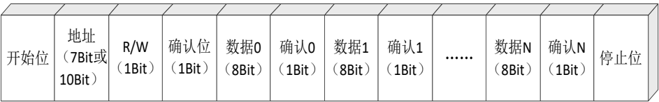
图3.133 I2C 帧格式
