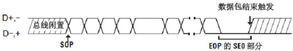
图3.242 USB 帧格式
