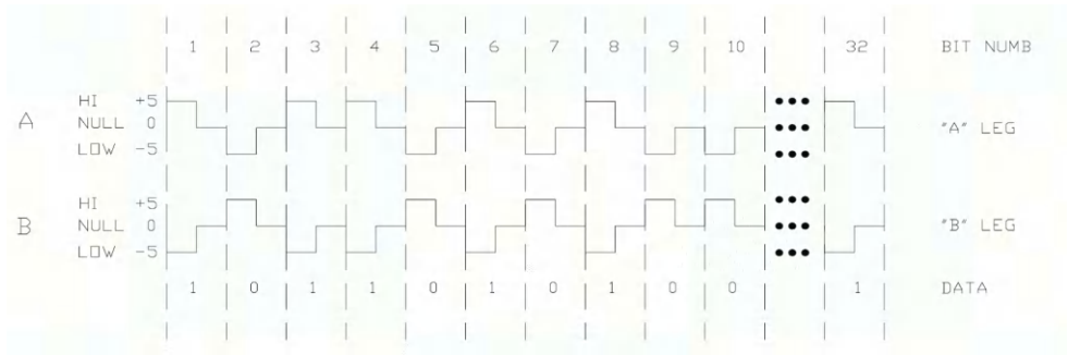
图3.274 ARINC 429 信号格式
