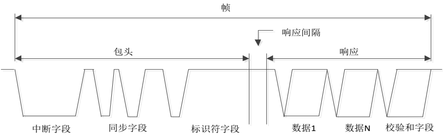
图3.191 LIN 帧格式
