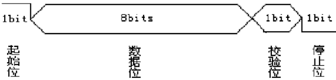
图3.150 RS232 帧格式
