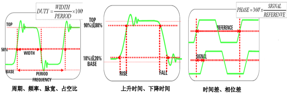
图3.49 时间参数
