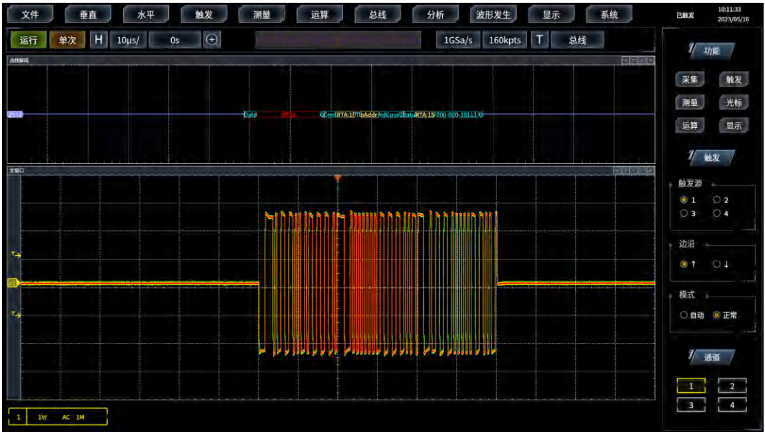
图3.273 MIL-STD-1553 触发与分析示例
