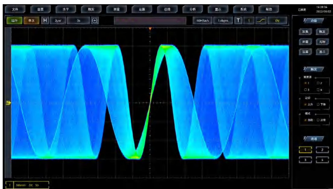
数字内插技术，实现触发点准确定位
