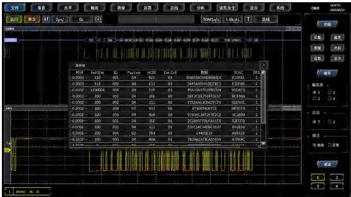
多种视图显示：数字视图、总线视图及事件表
