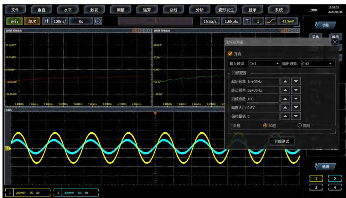
波特图分析（选件 S03）：检测控制环路的频率响应，分析反馈系统的稳定性
