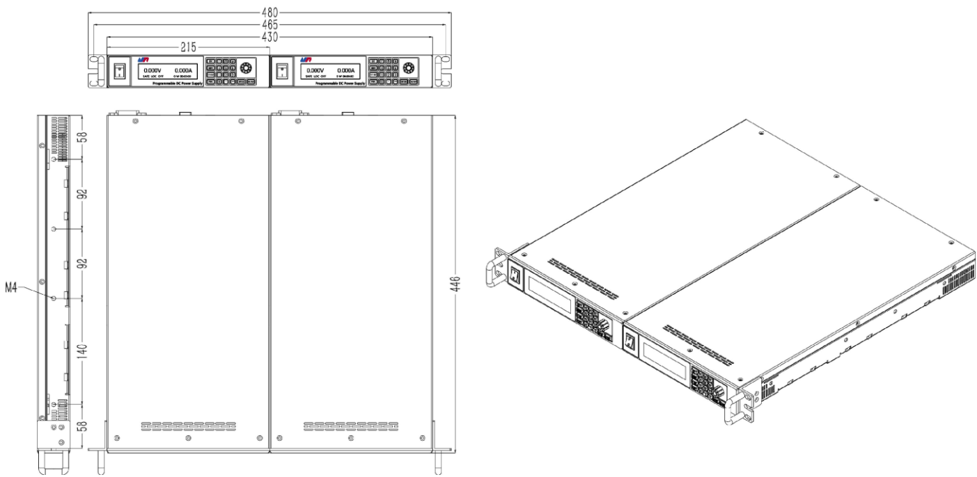
两台 DM 机型 19 英寸标准机柜安装尺寸图
