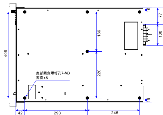
IPX-S系列 10kW 中高压小电流尺寸 d示意图
