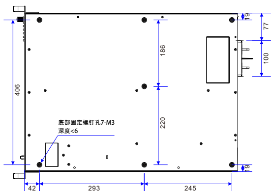
IPX-S系列 2~5kW 中高压小电流尺寸 b示意图
