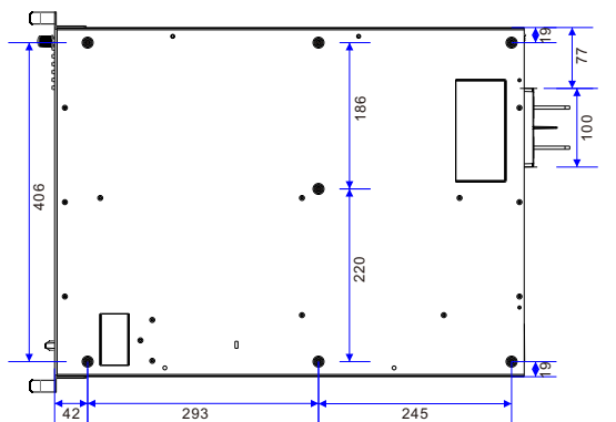
IPX-S系列 2~5kW 低压大电流尺寸 a示意图
