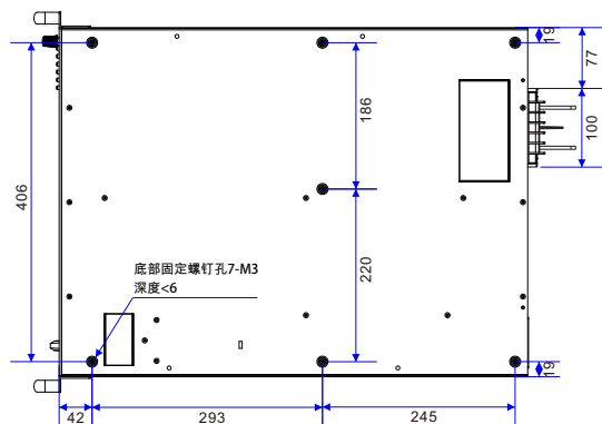
IPX-S系列 10kW 低压大电流尺寸 c示意图
