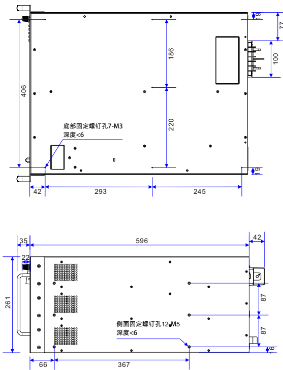
IPX-S系列 15kW 中高压小电流尺寸 f示意图
