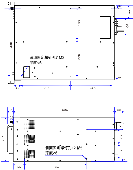
IPX-S系列 15kW 低压大电流尺寸 e示意图
