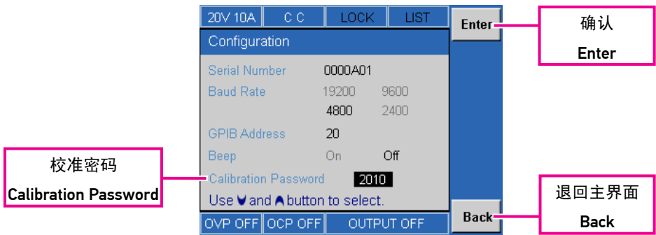
图 4-9 Config 参数设置界面
