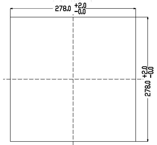
安装开孔尺寸 278×278mm
