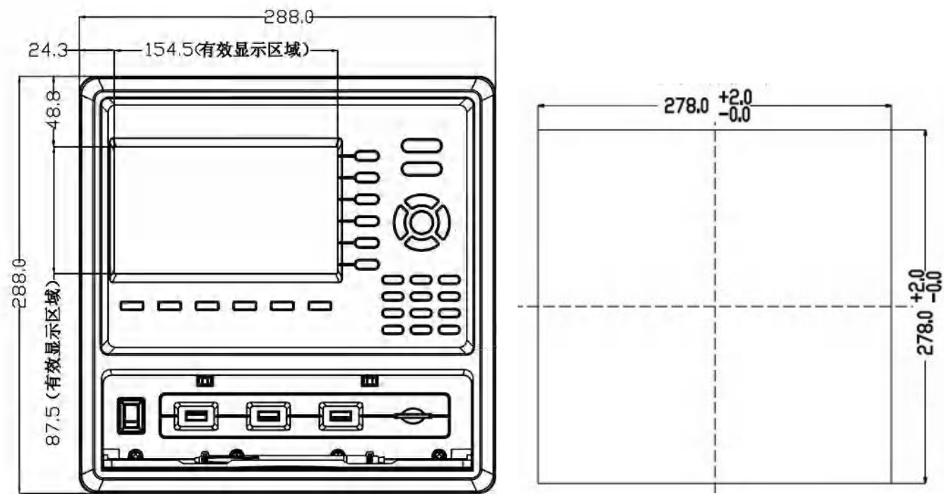
外形尺寸：288×288×200mm (长×宽×深)
